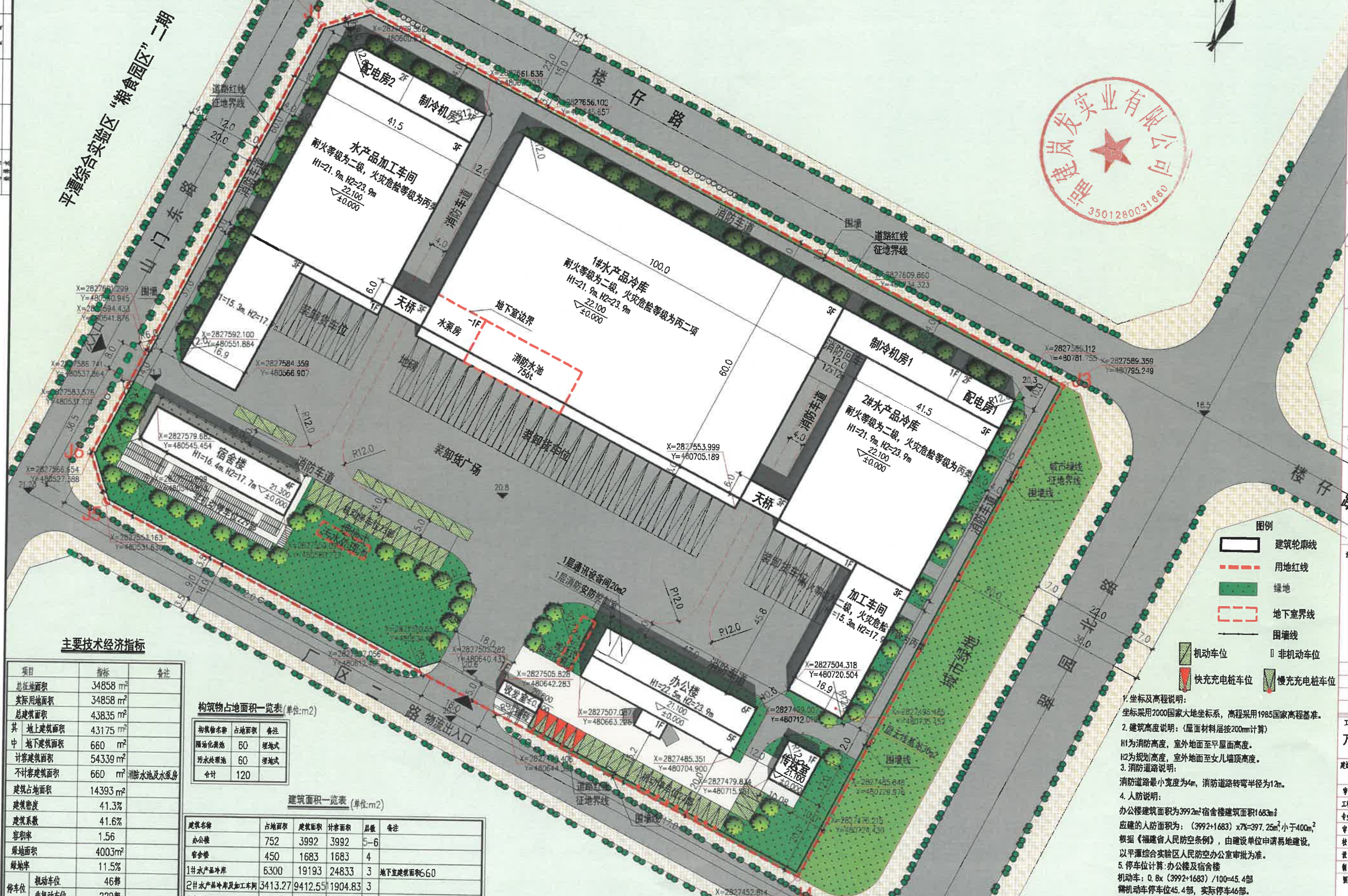
拟变更总平面图 1:500
