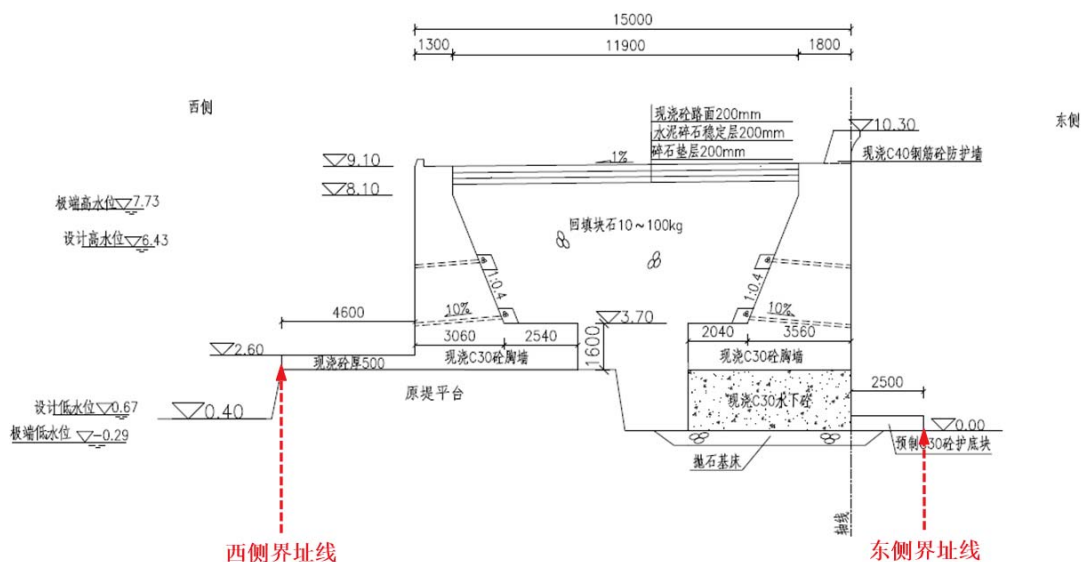
防波堤结构断面图2-2
