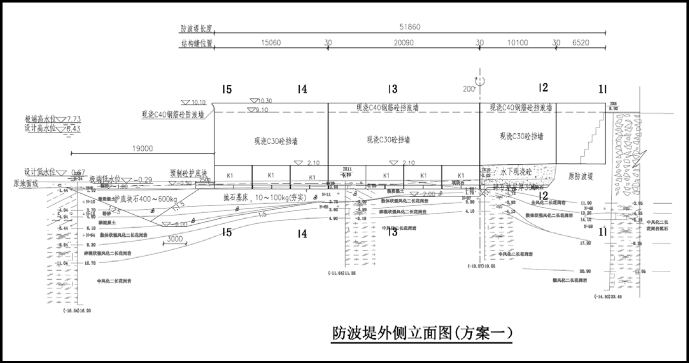
图 2.2-8 本项目防波堤延长段立面图
