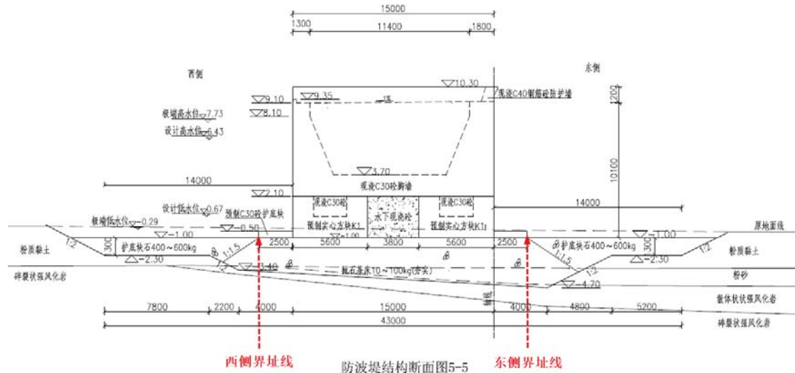
图 7.3-3 本项目界址线确定依据（断面 4-4~断面 5-5 之间）
