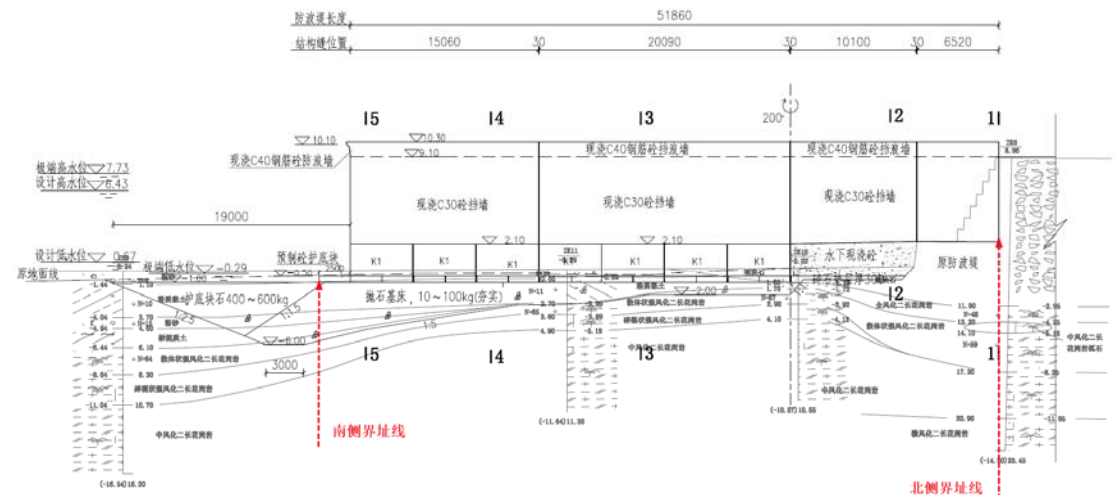
防波堤外侧立面图(方案一)
