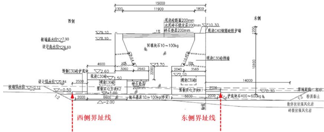
防波堤结构断面图3-3
