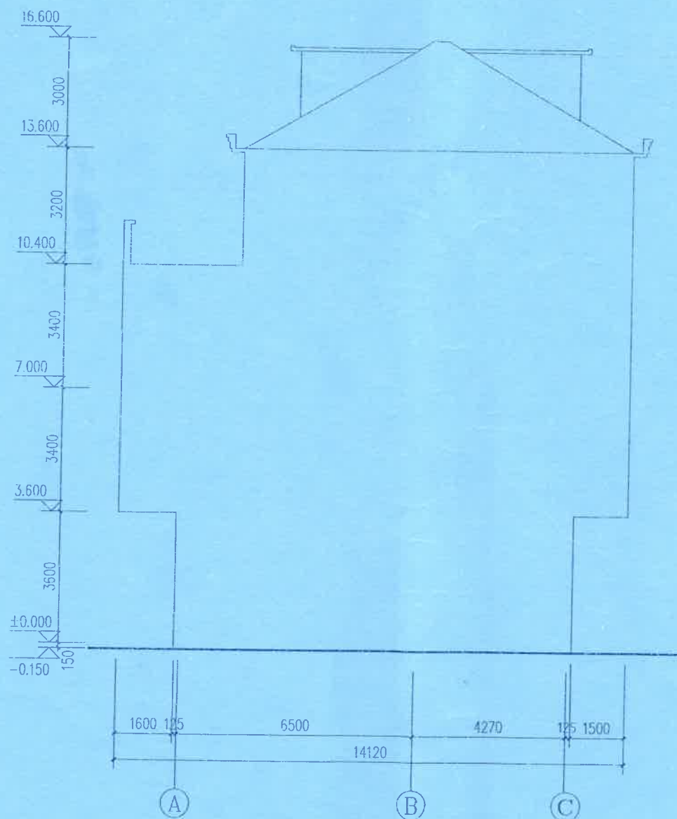
A~C轴立面图 1:100
