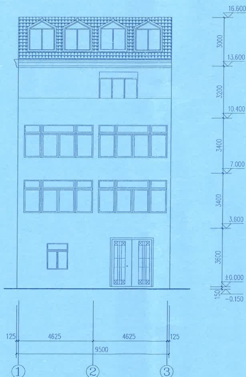
①~③轴立面图 1:100
