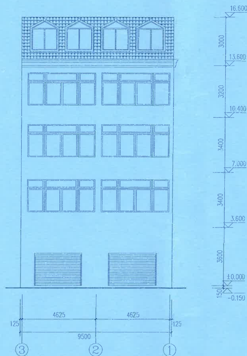
③~①轴立面图 1:100 (沿街面)
