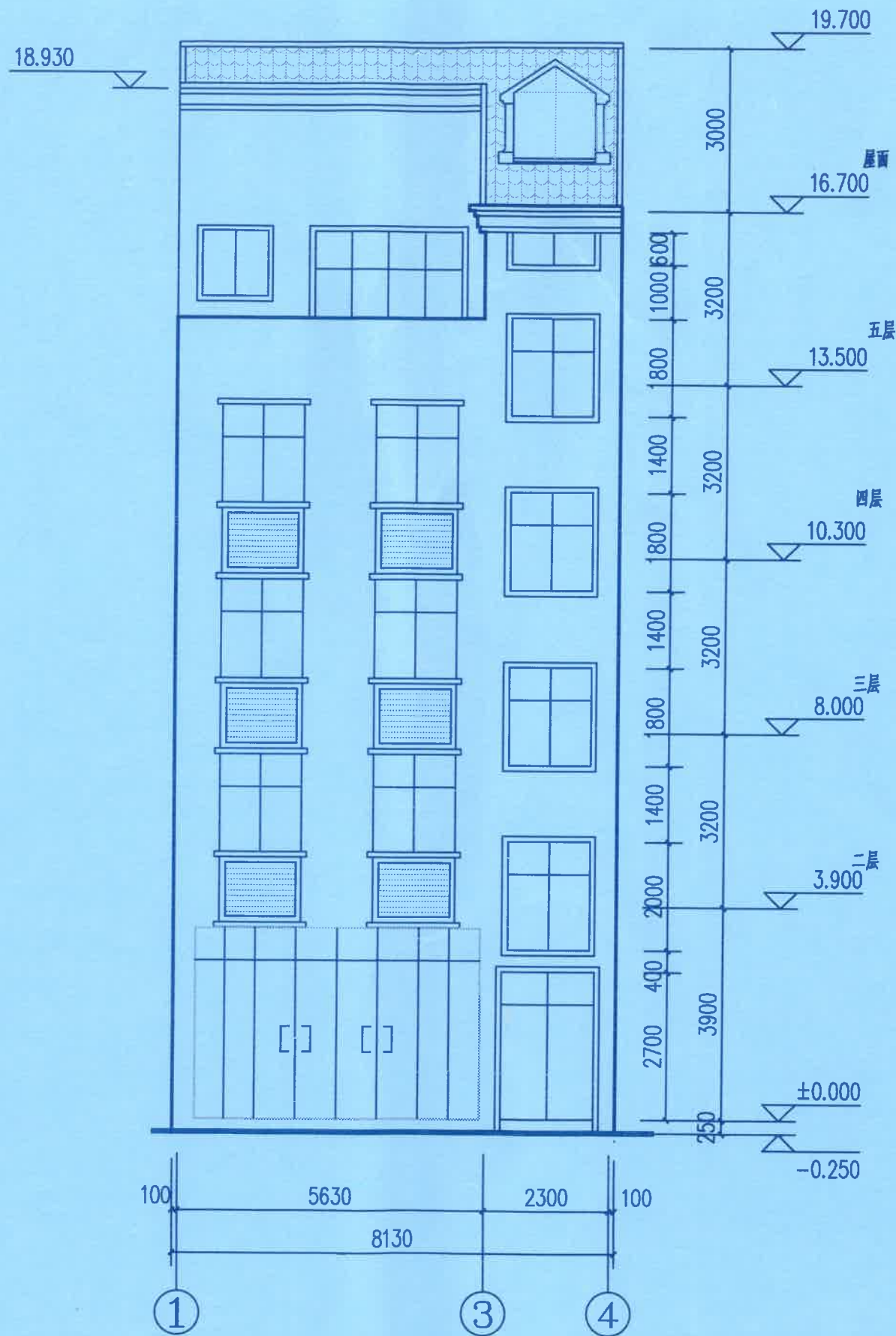
①~④轴立面图 1:100
