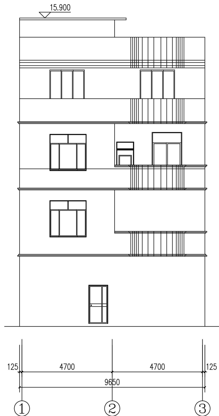
①~③轴立面图 1:100
