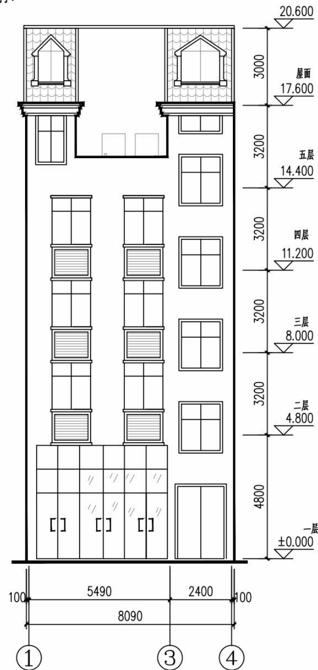
变更前①~④轴立面图 1:100 (北立面)
