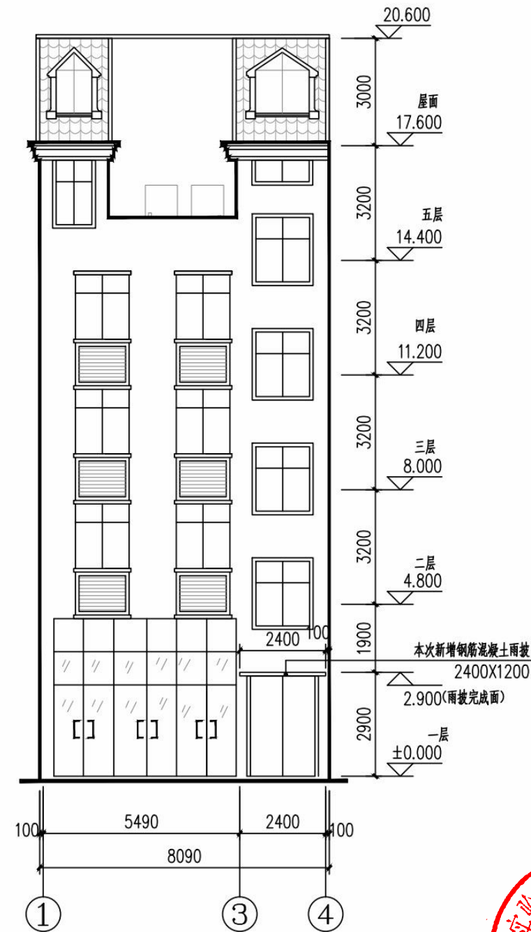
变更后①~④轴立面图 1:100 (北立面)
