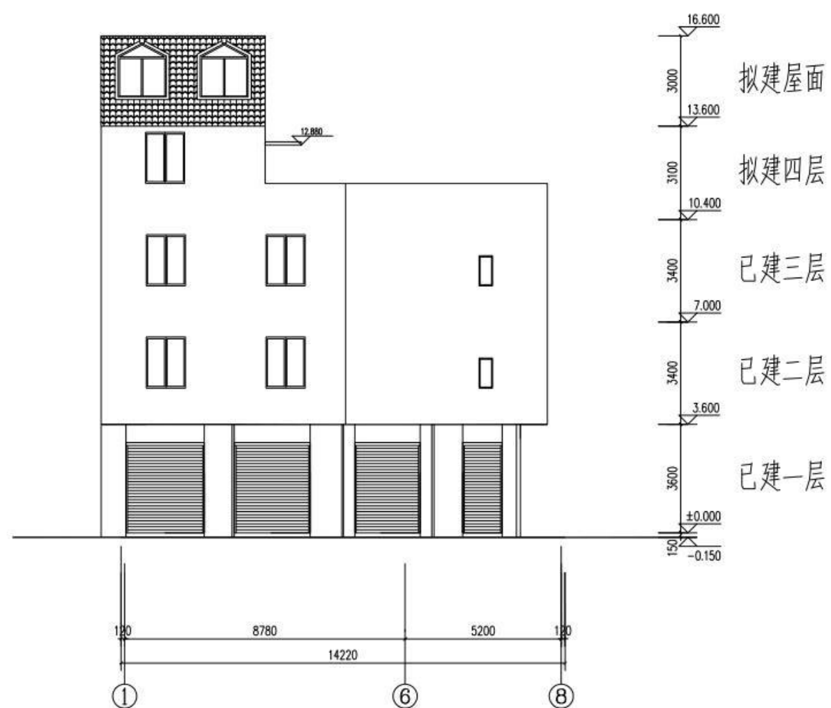
①~⑧轴立面图 1:100
