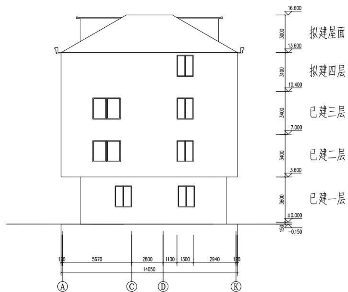
A~K轴立面图 1:100
