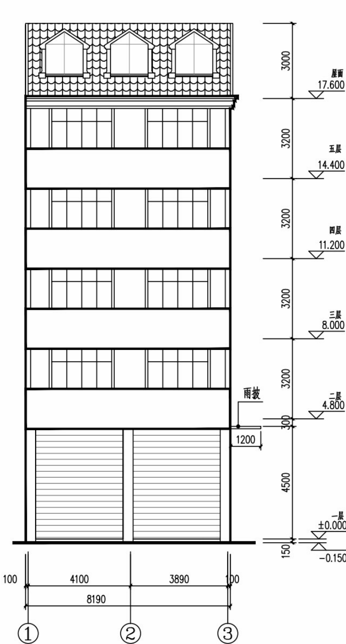
①~③轴立面图 1:100 (沿街面·南立面)
