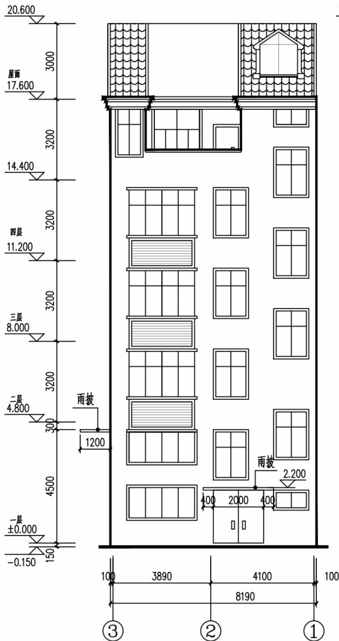
③~①轴立面图 1:100 (北立面)
