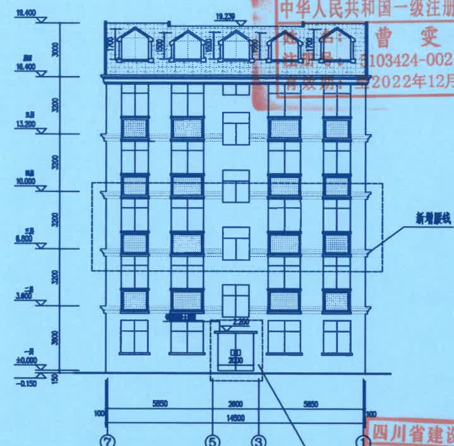
⑦~①轴立面图 1:100 (北立面)
