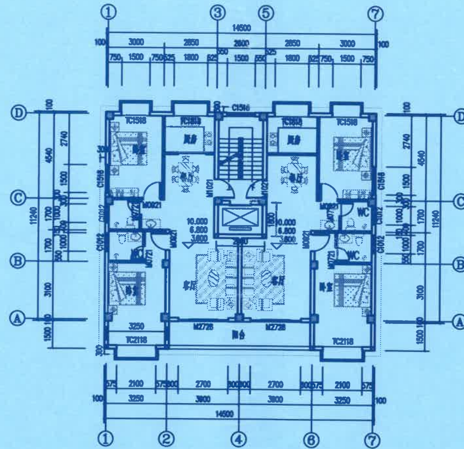
二至四层平面图 1:100
