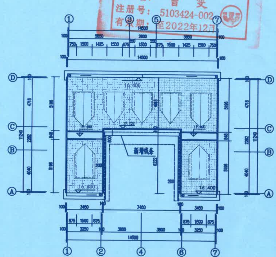
屋面平面图 1:100
