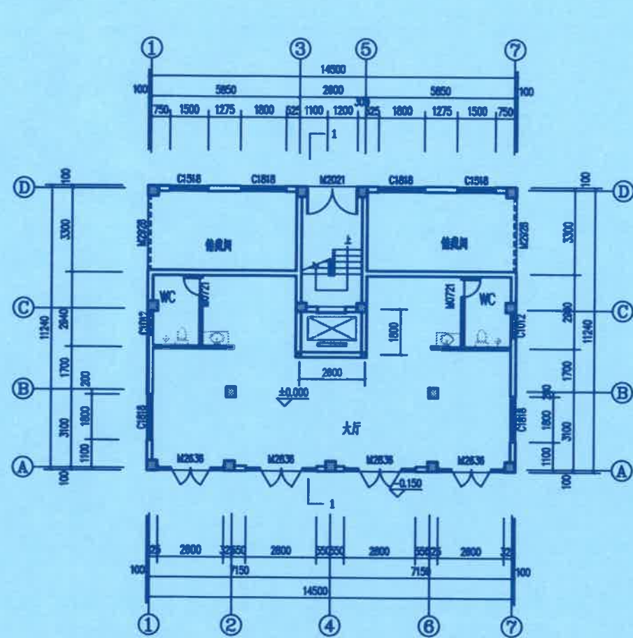
一层平面图 1:100
