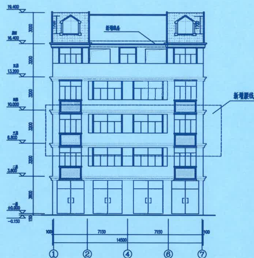
①~⑦轴立面图 1:100 (南立面)
