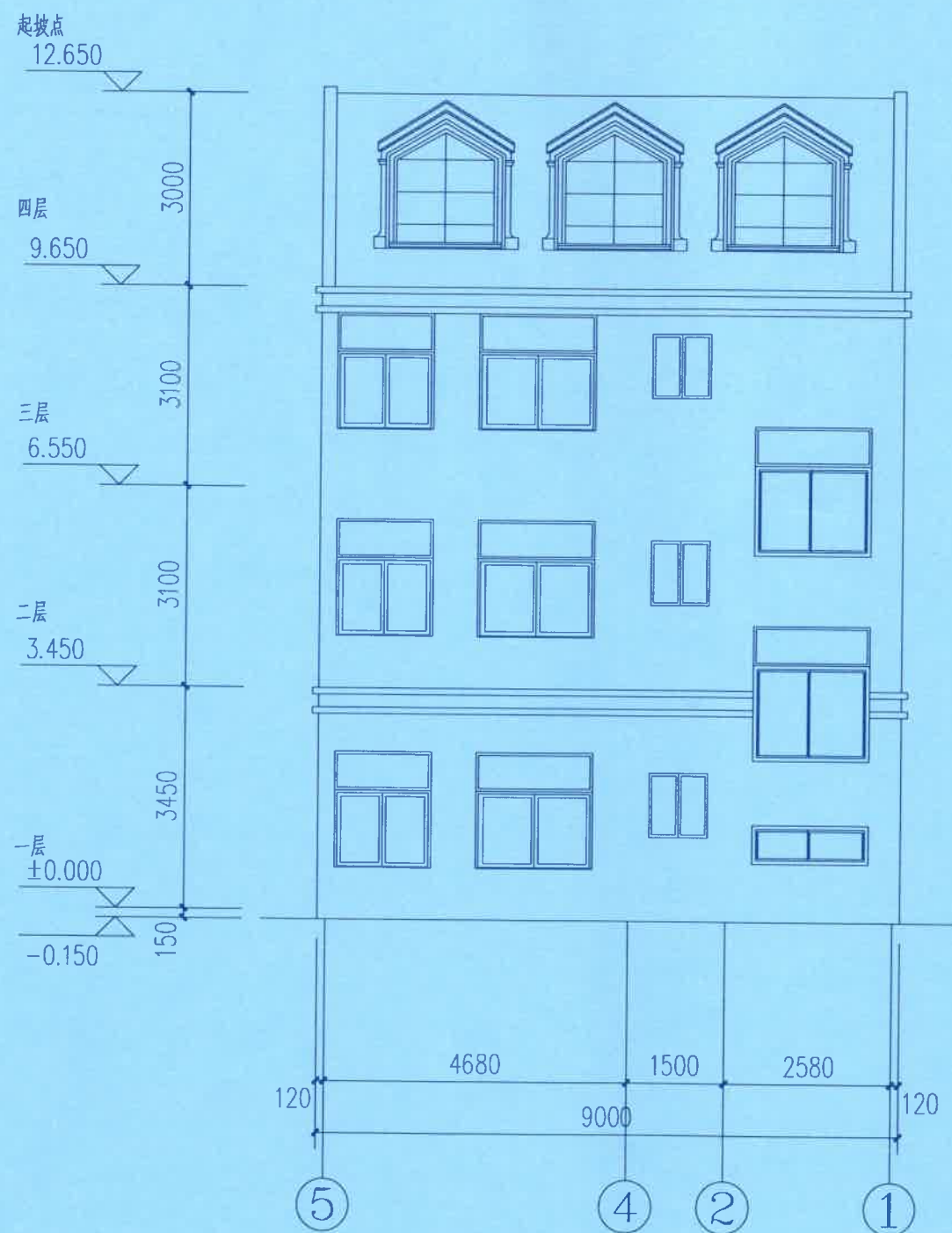
⑤-①轴立面图 1:100
