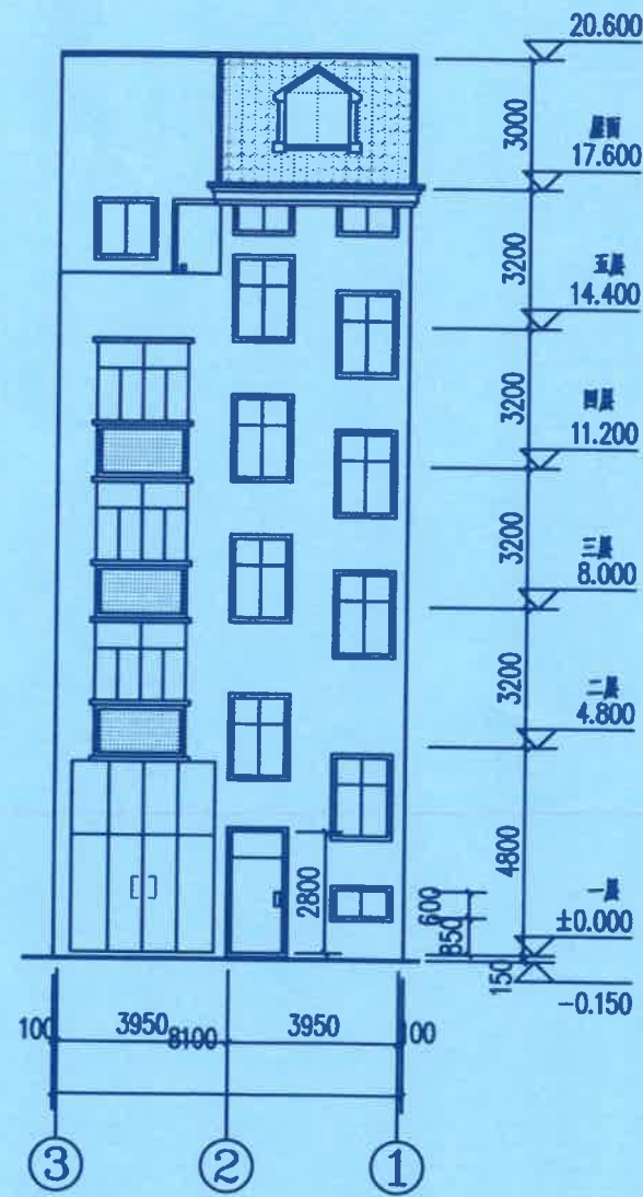
③~①轴变更前立面图 1:100 (北立面)
