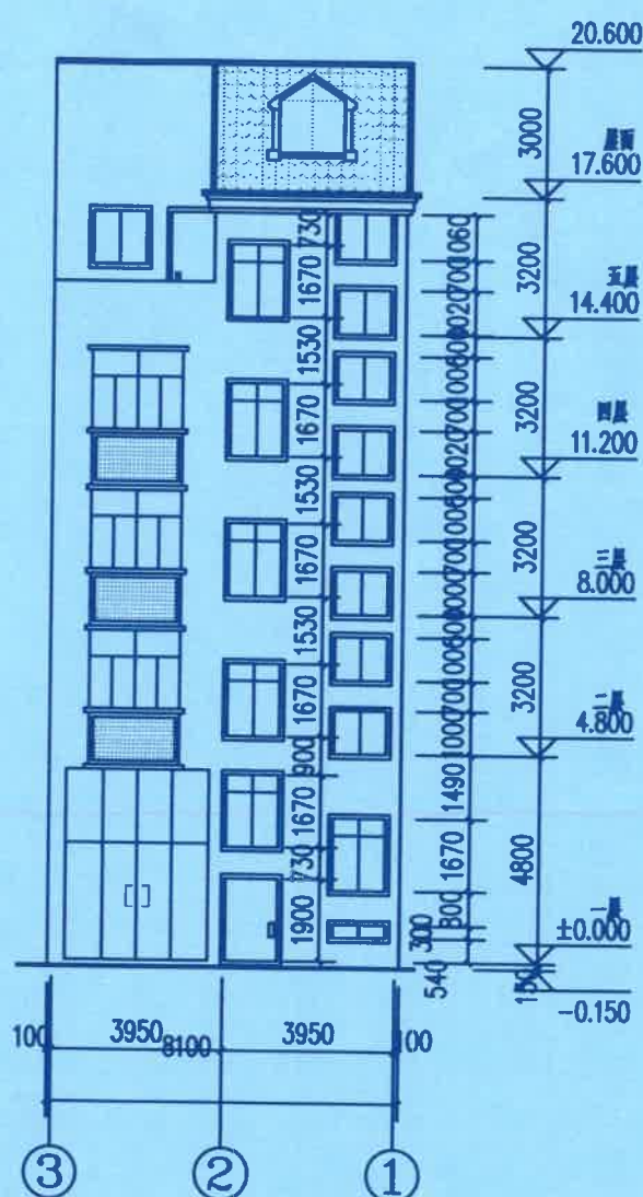
③~①轴变更后立面图 1:100 (北立面)
