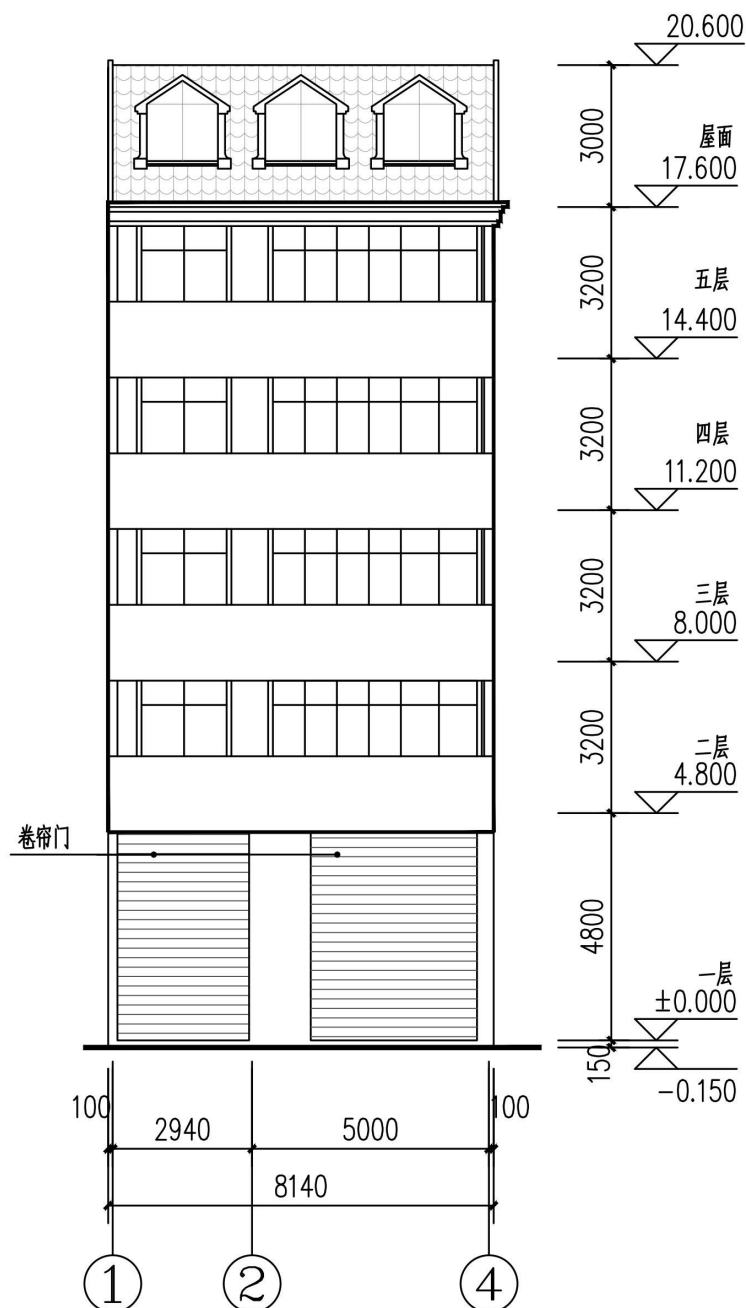
①~④轴立面图 1:100 (沿街立面·西立面)
