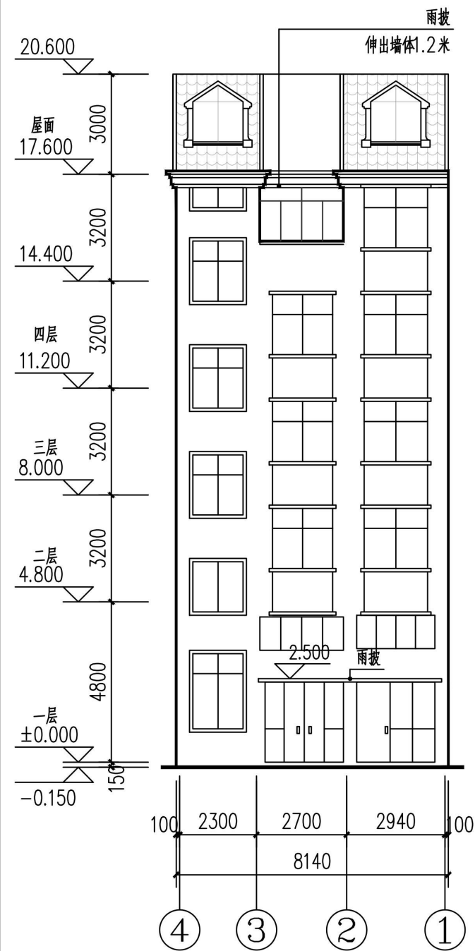
④~①轴立面图 1:100 (背立面·东立面)
