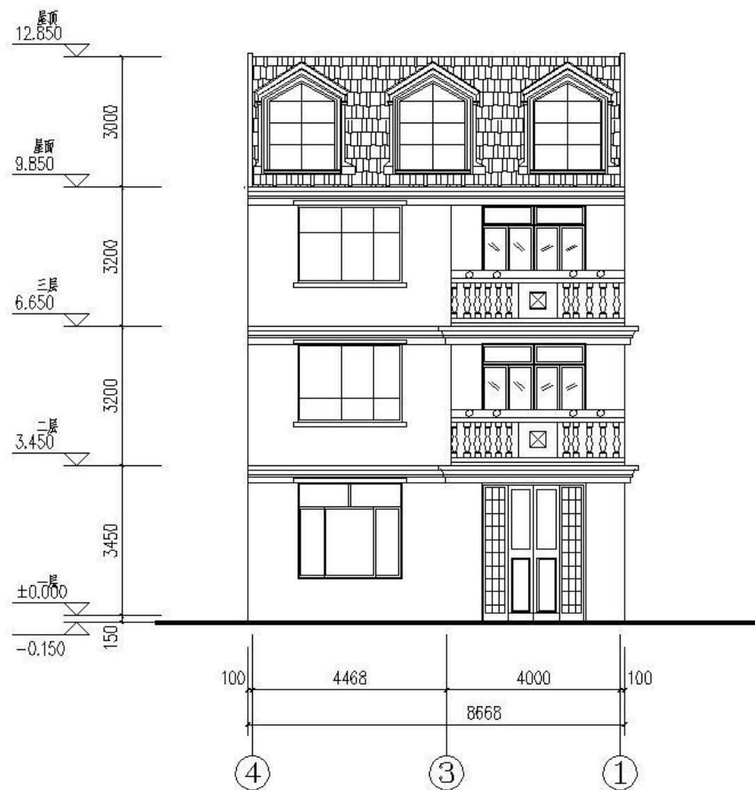
① - ④ 轴立面图 1:100 (变更前)
