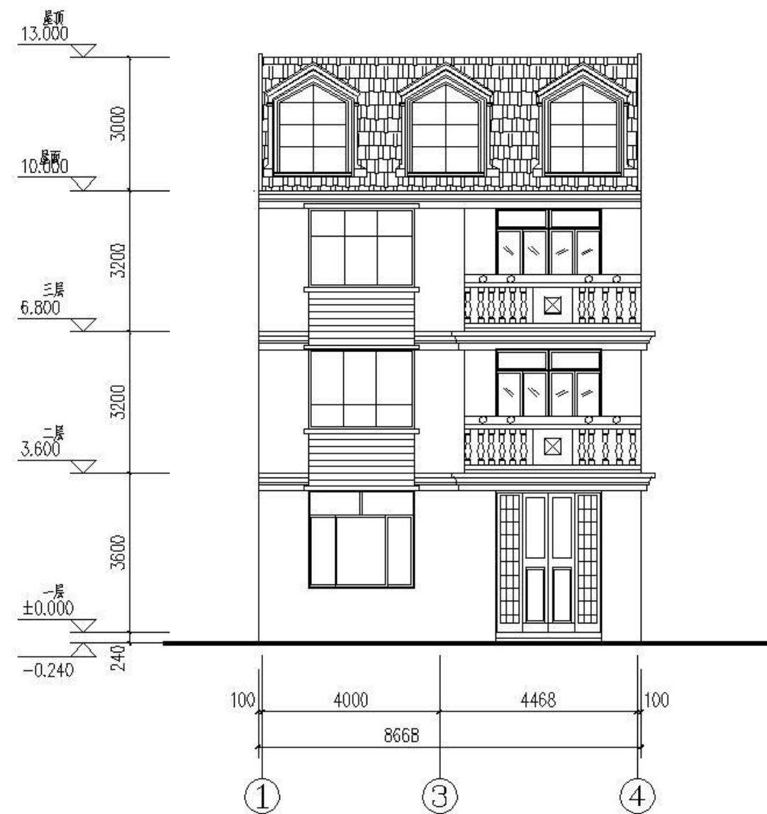
① ④ 轴立面图 1:100 (变更后)
