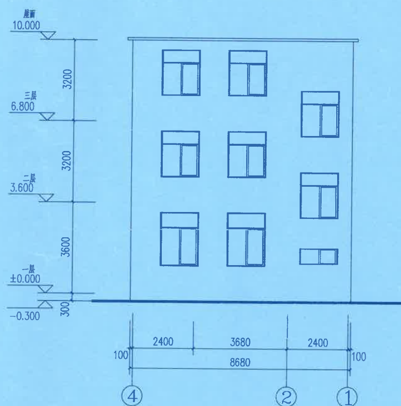
④ - ① 轴立面图 1:100
