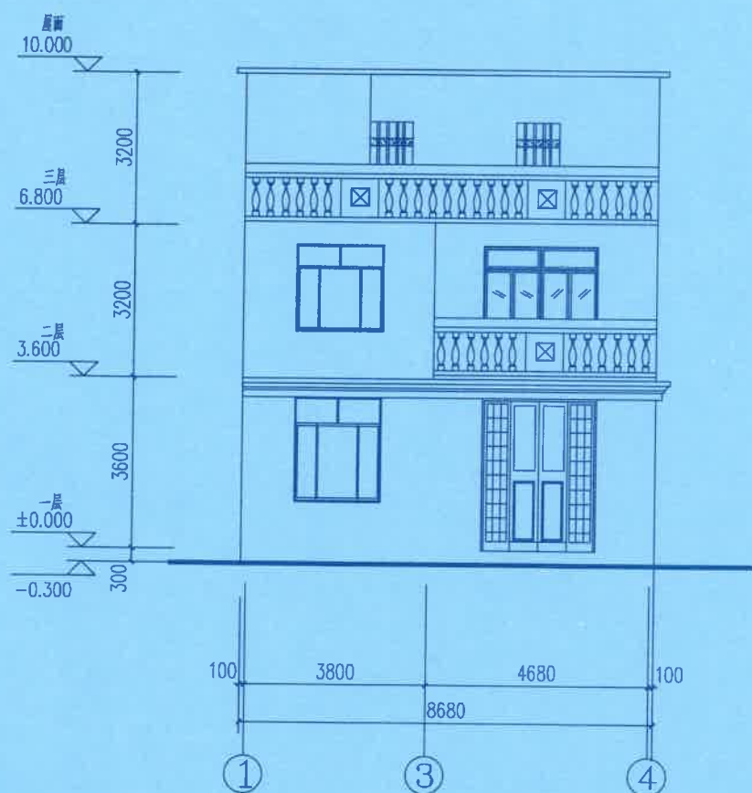
① - ④ 轴立面图 1:100
