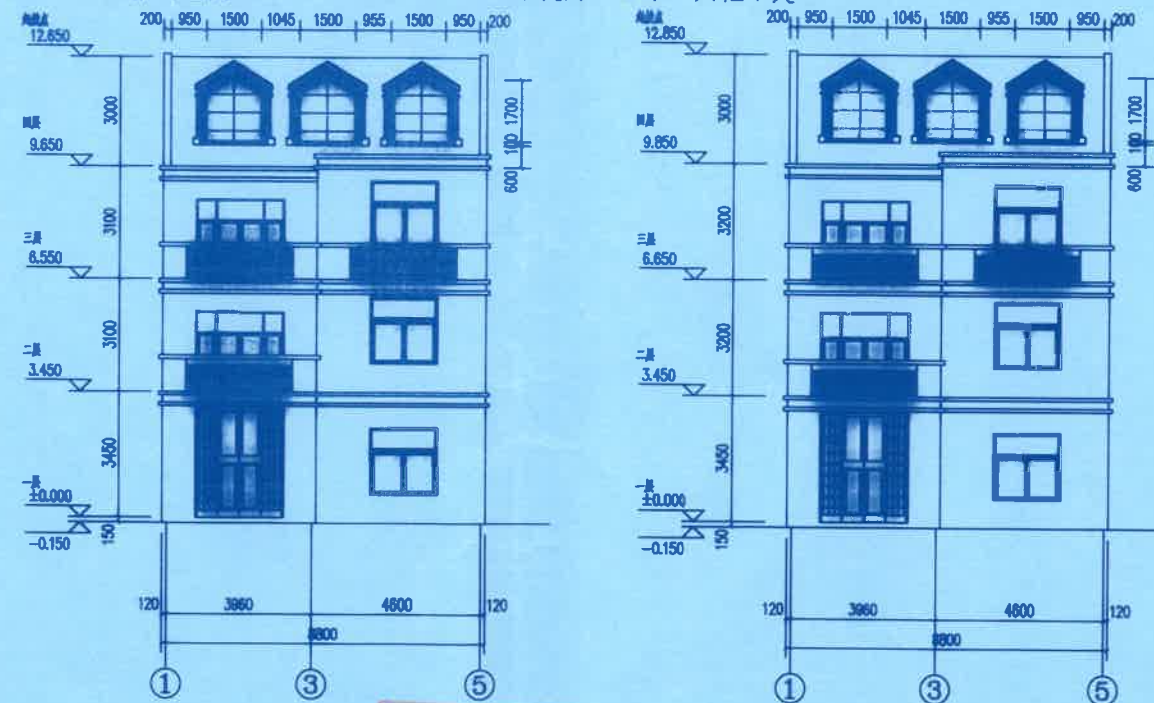
①~⑤轴立面图 1:100 (变更前)
