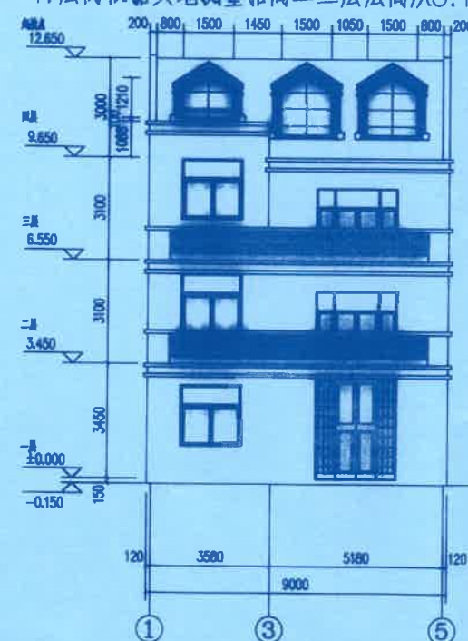
①~⑤轴立面图 1:100 (变更前)
