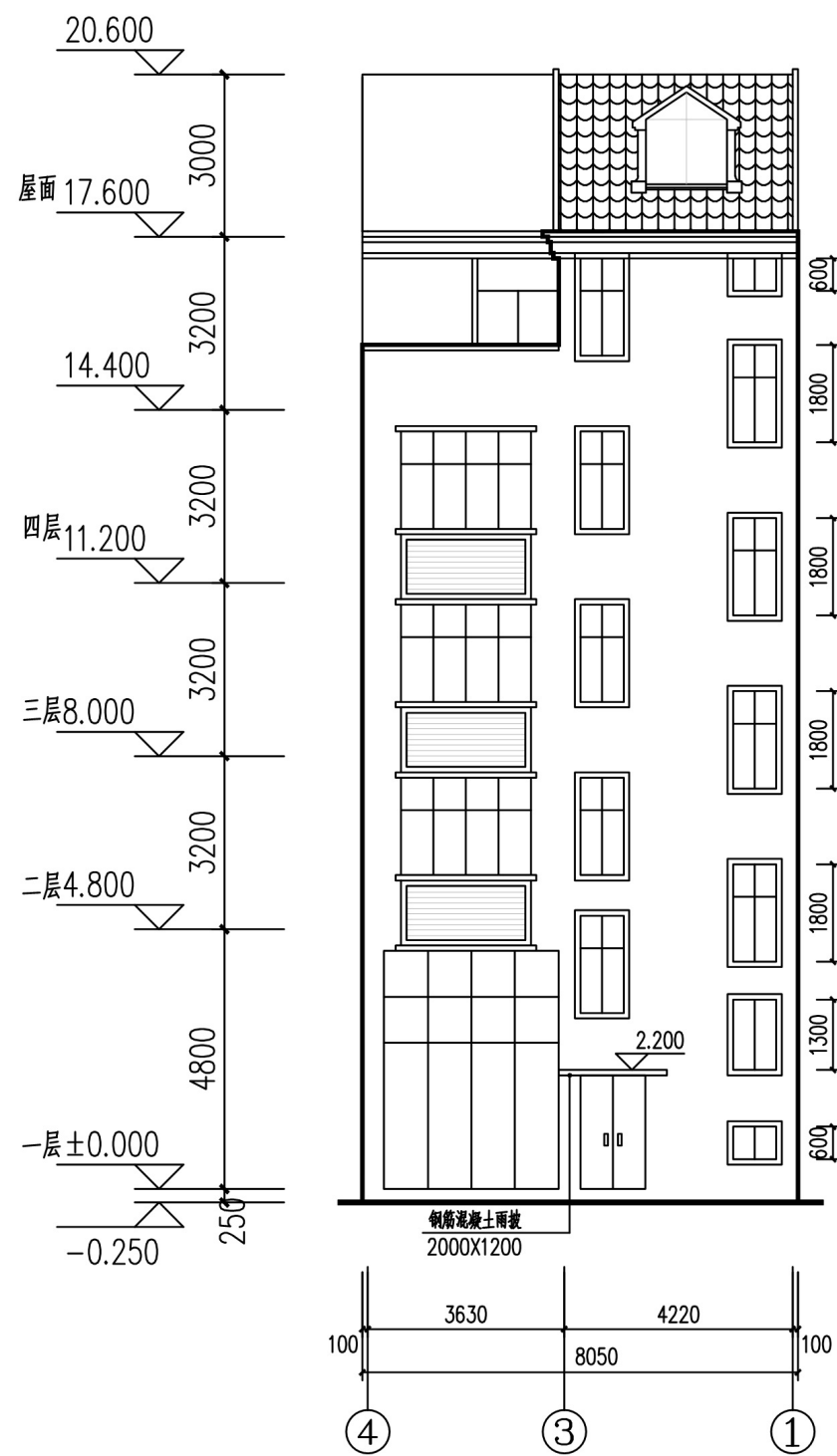
④~①轴立面图 1:100 (背立面·北立面)
