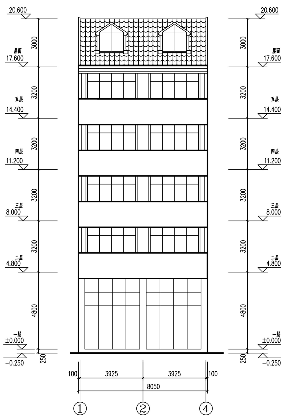
①~④轴立面图 1:100 (沿街面·南立面)
