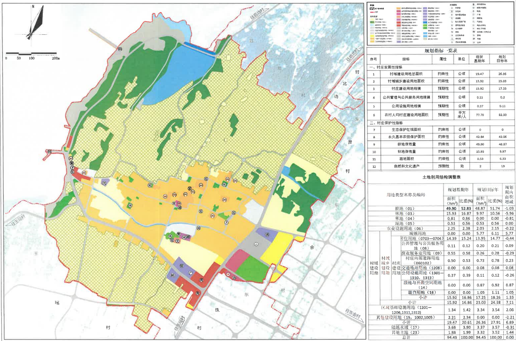
村域综合规划图
