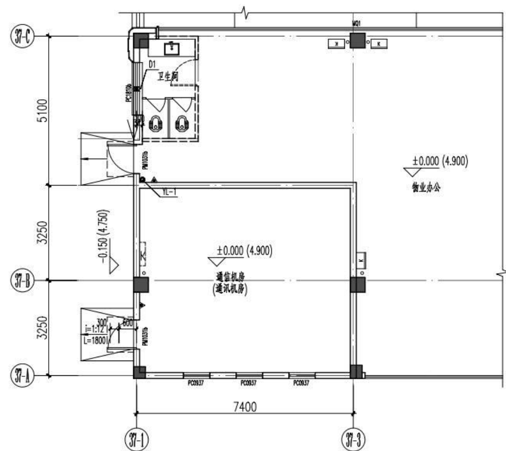
37号楼原一层局部平面图
