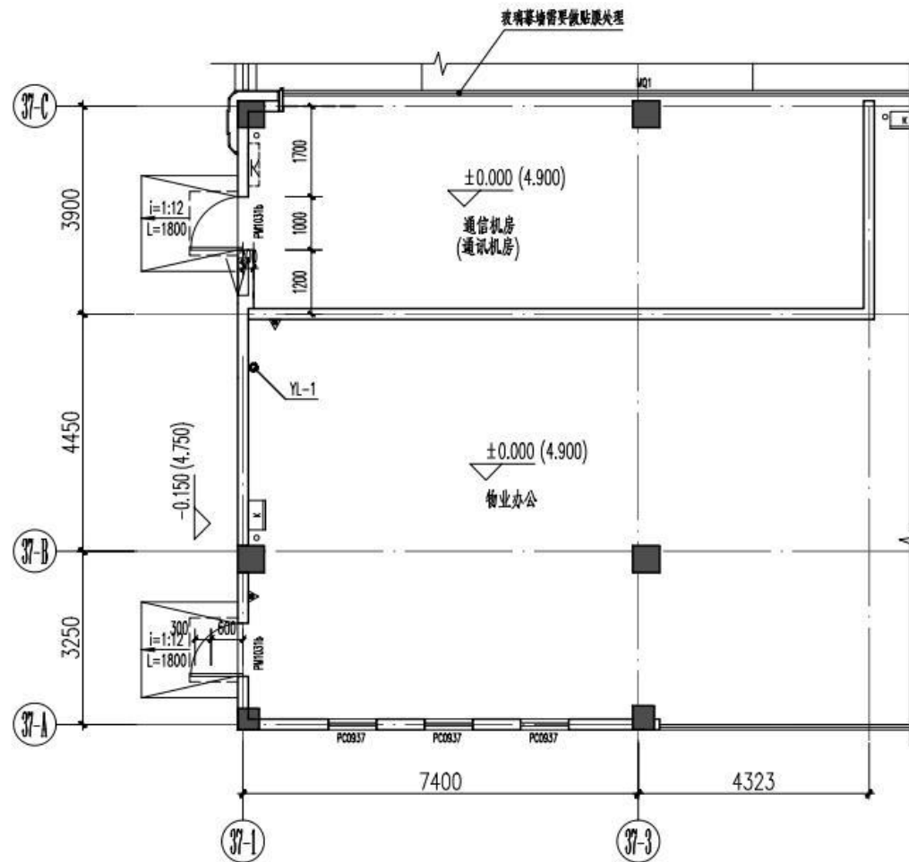
37号楼修改后一层局部平面图
