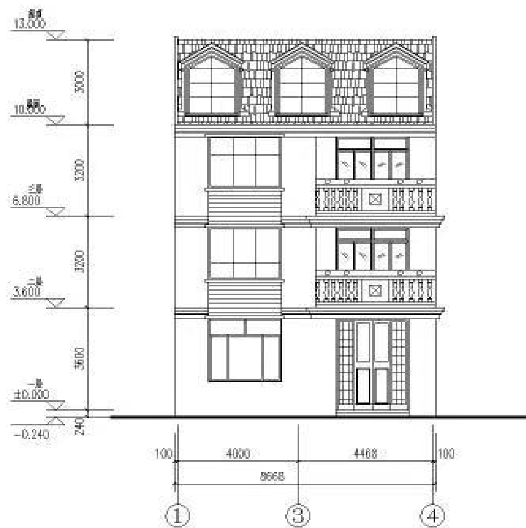
① - ④ 轴立面图 1:100
