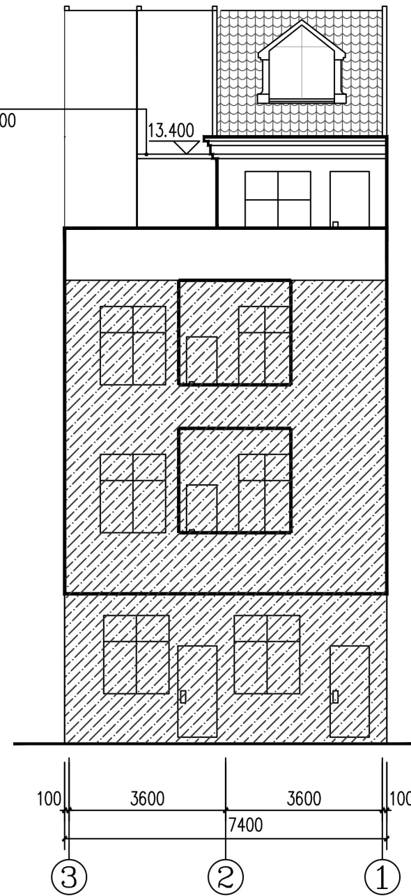
③~①轴立面图 1:100
