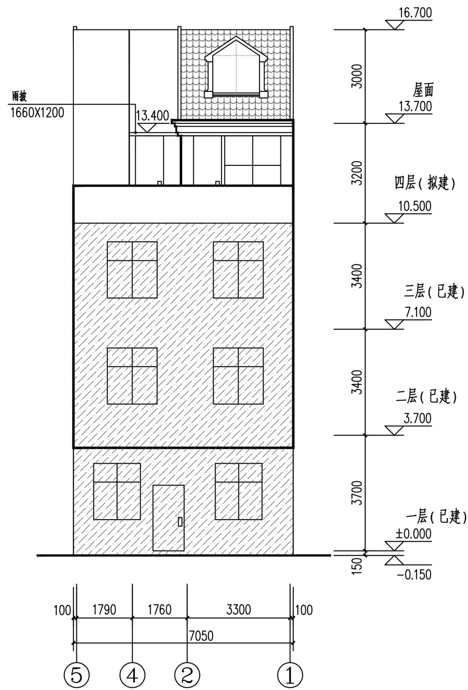
⑤~①轴立面图 1:100
