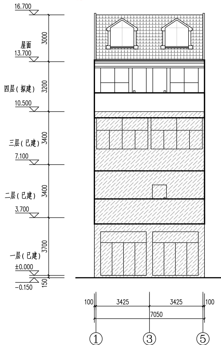
①~⑤轴立面图 1:100 (沿街立面)
