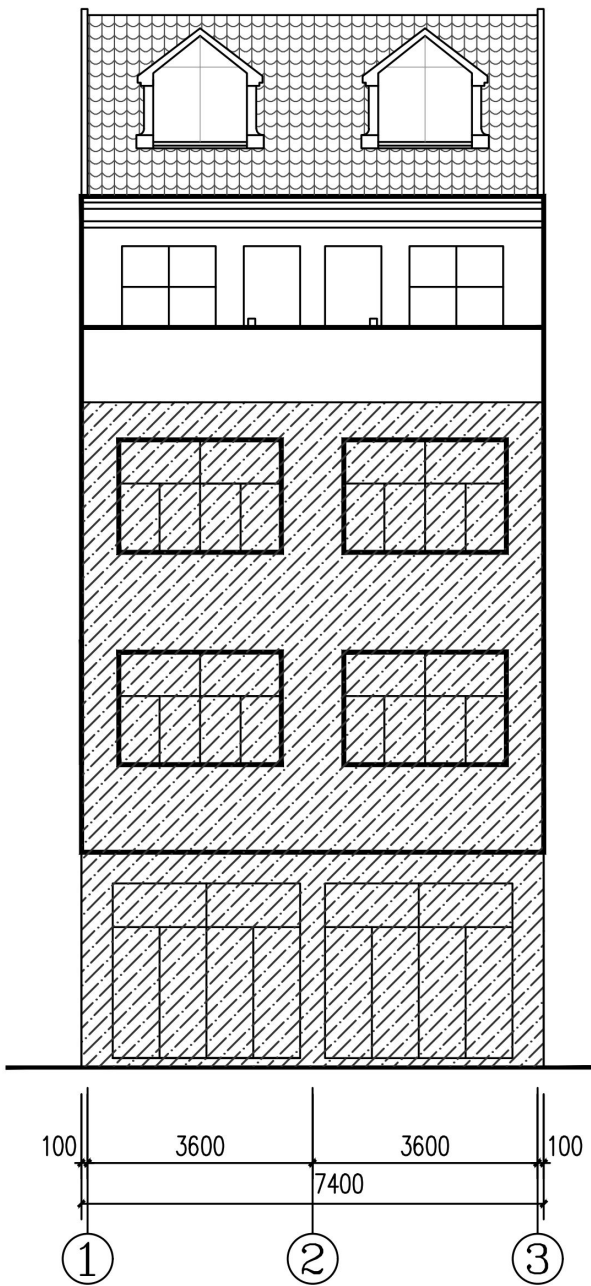
①~③轴立面图 1:100 (沿街面)
