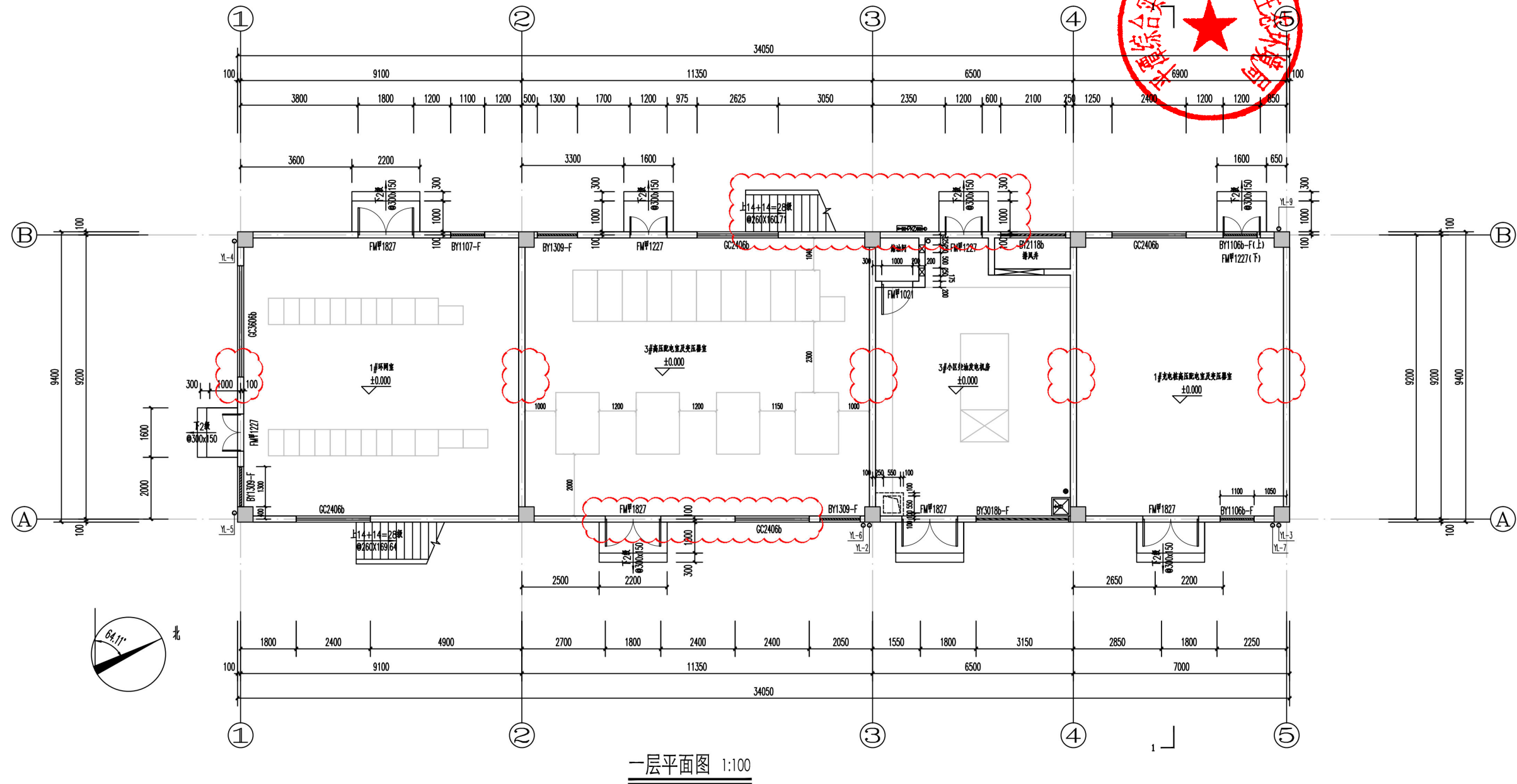
附图2：平面调整前
