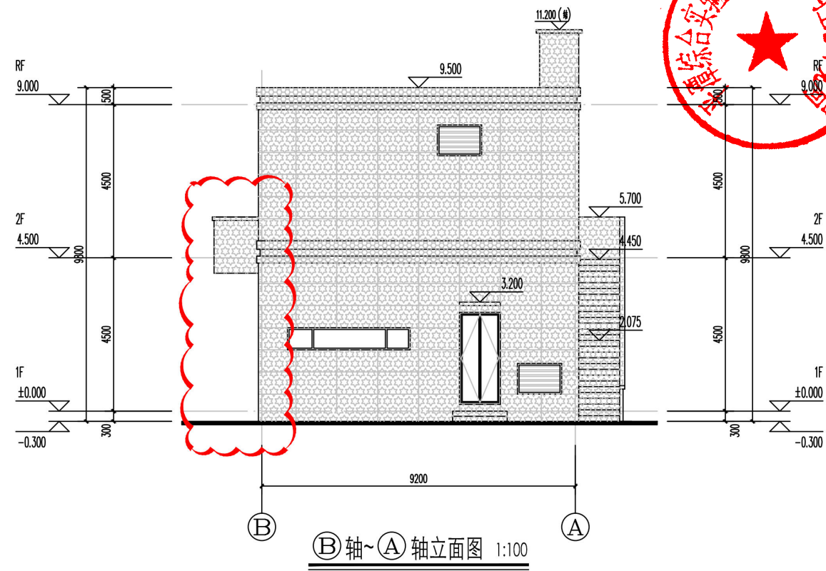
附图9：立面调整后
