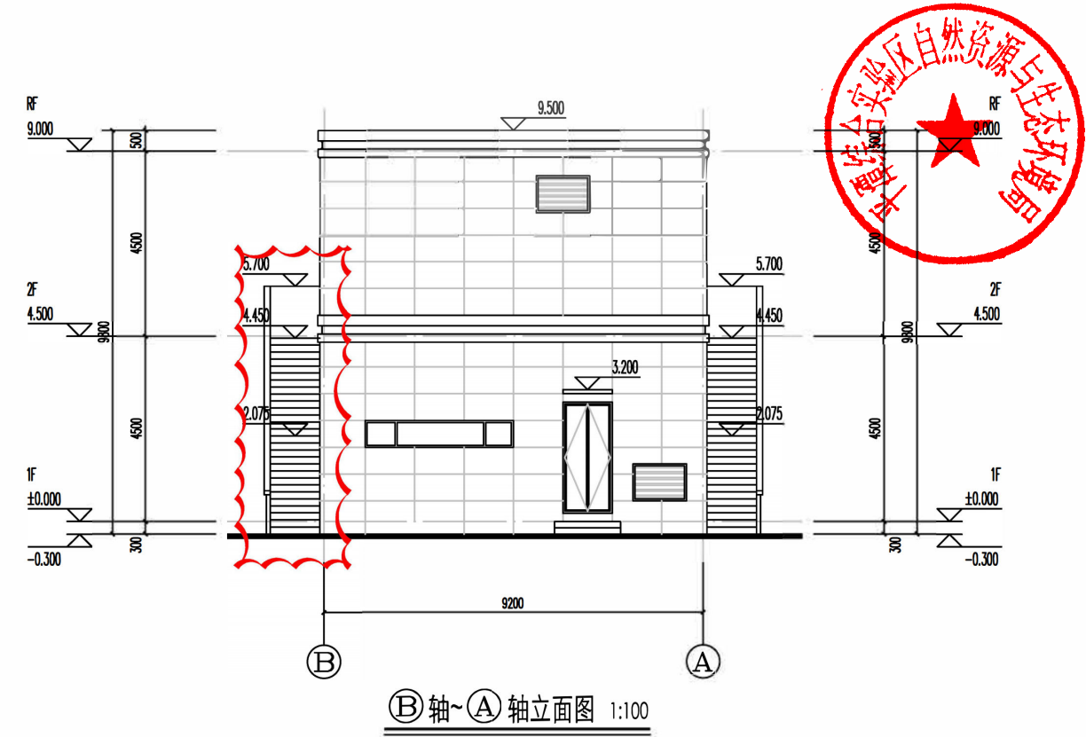
附图7：立面调整前
