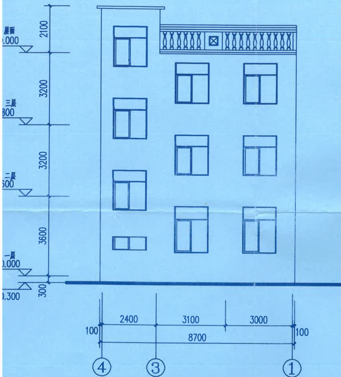
④-①轴立面图 1:100
