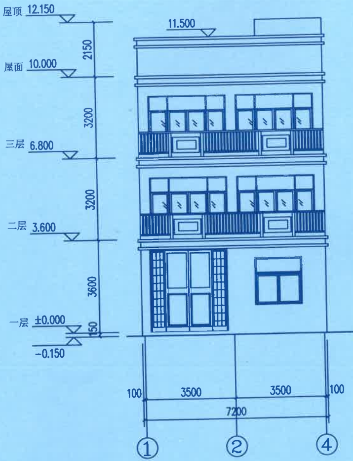
①-④ 轴立面图 1:100
