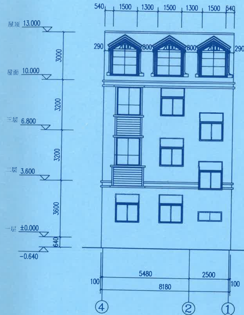
④-① 轴立面图 1:100
