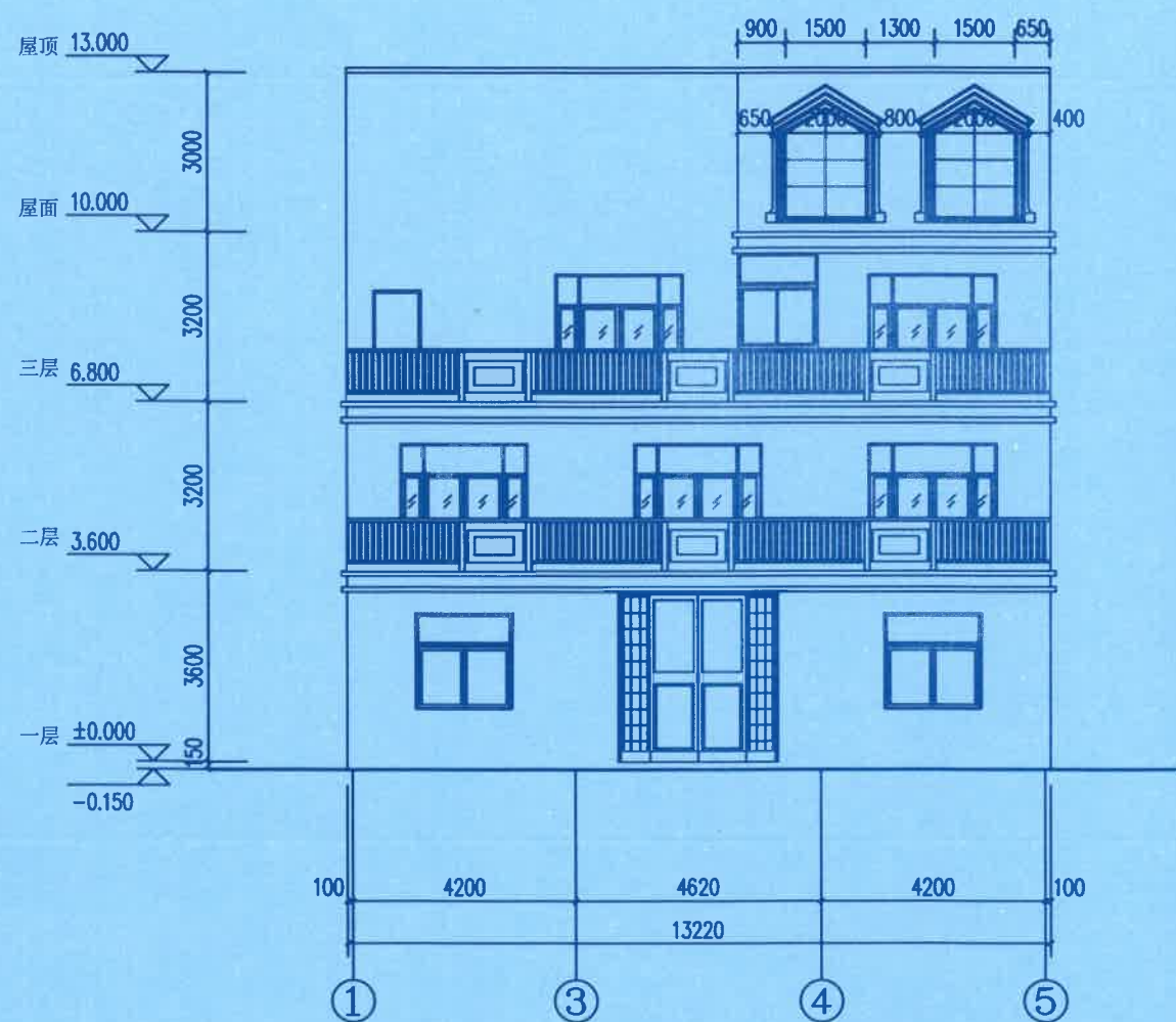
① - ⑤ 轴立面图 1:100
