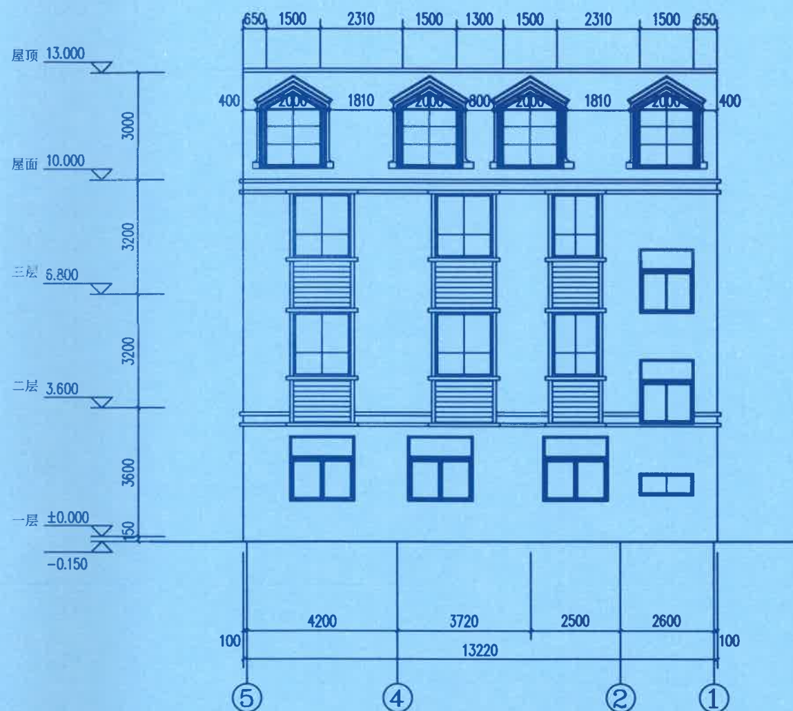
⑤-①轴立面图 1:100
