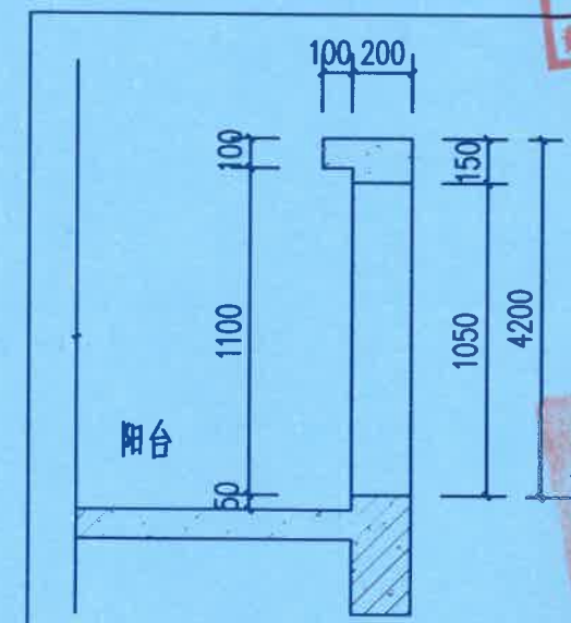
① 阳台大样详图 1:25
