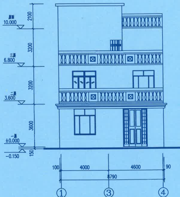
①-④ 轴立面图 1:100
