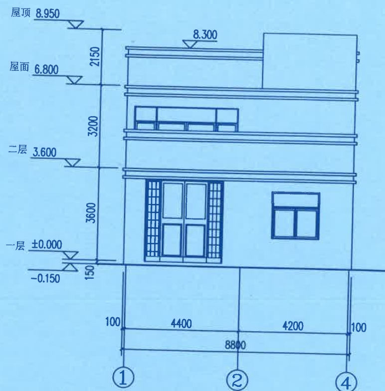
①-④轴立面图 1:100
