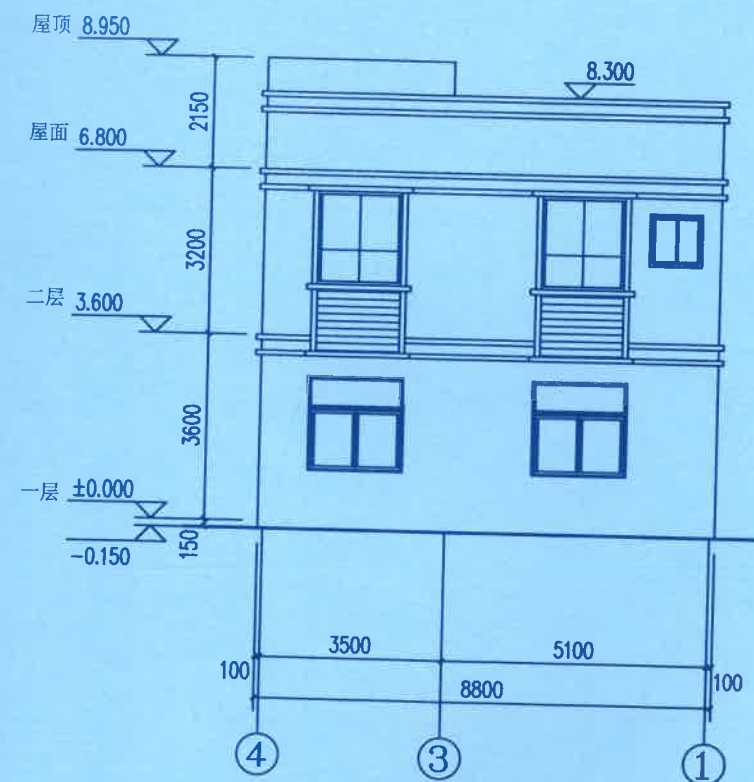
④-①轴立面图 1:100
