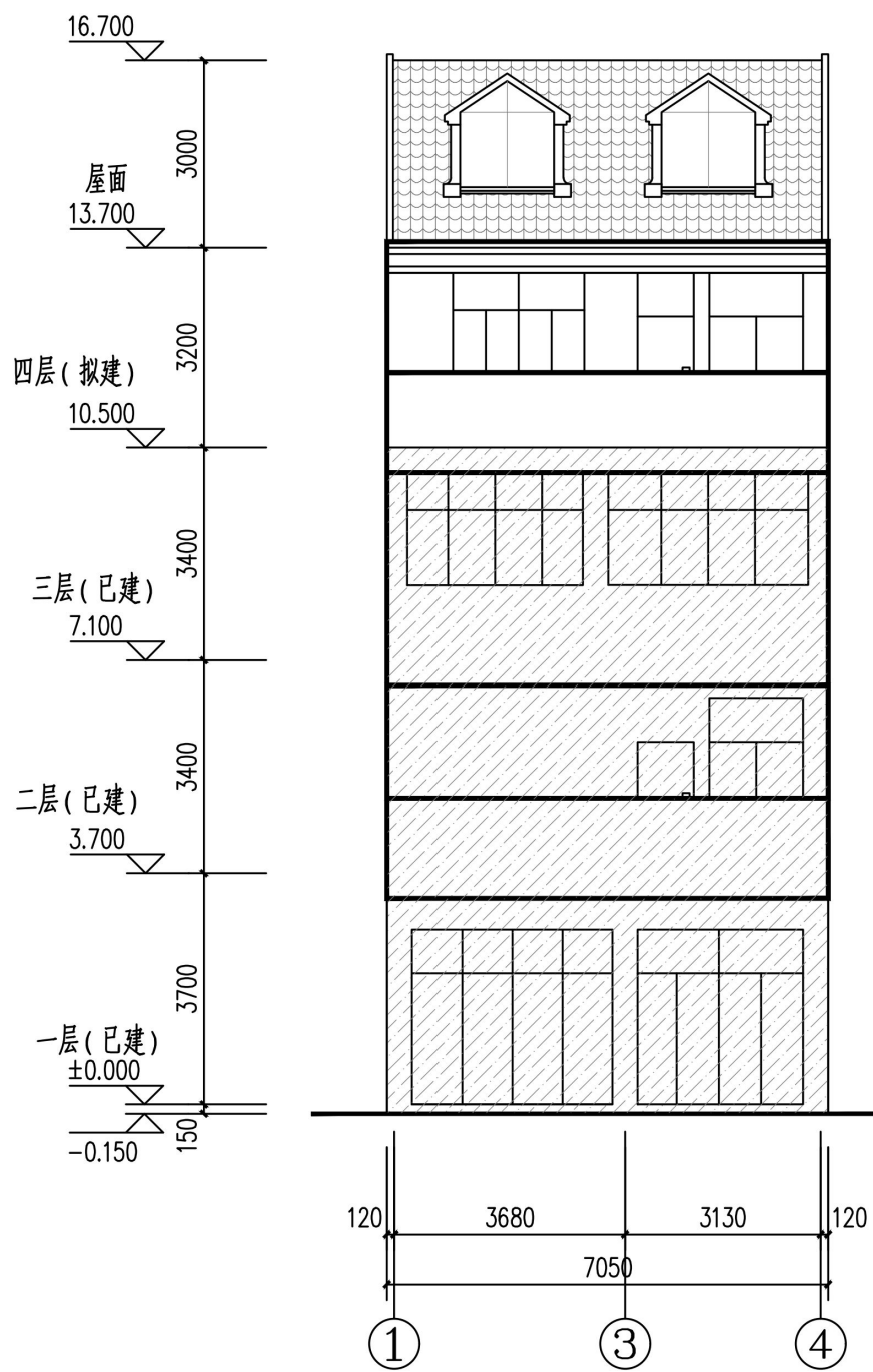
①~④轴立面图 1:100 (沿街面)
