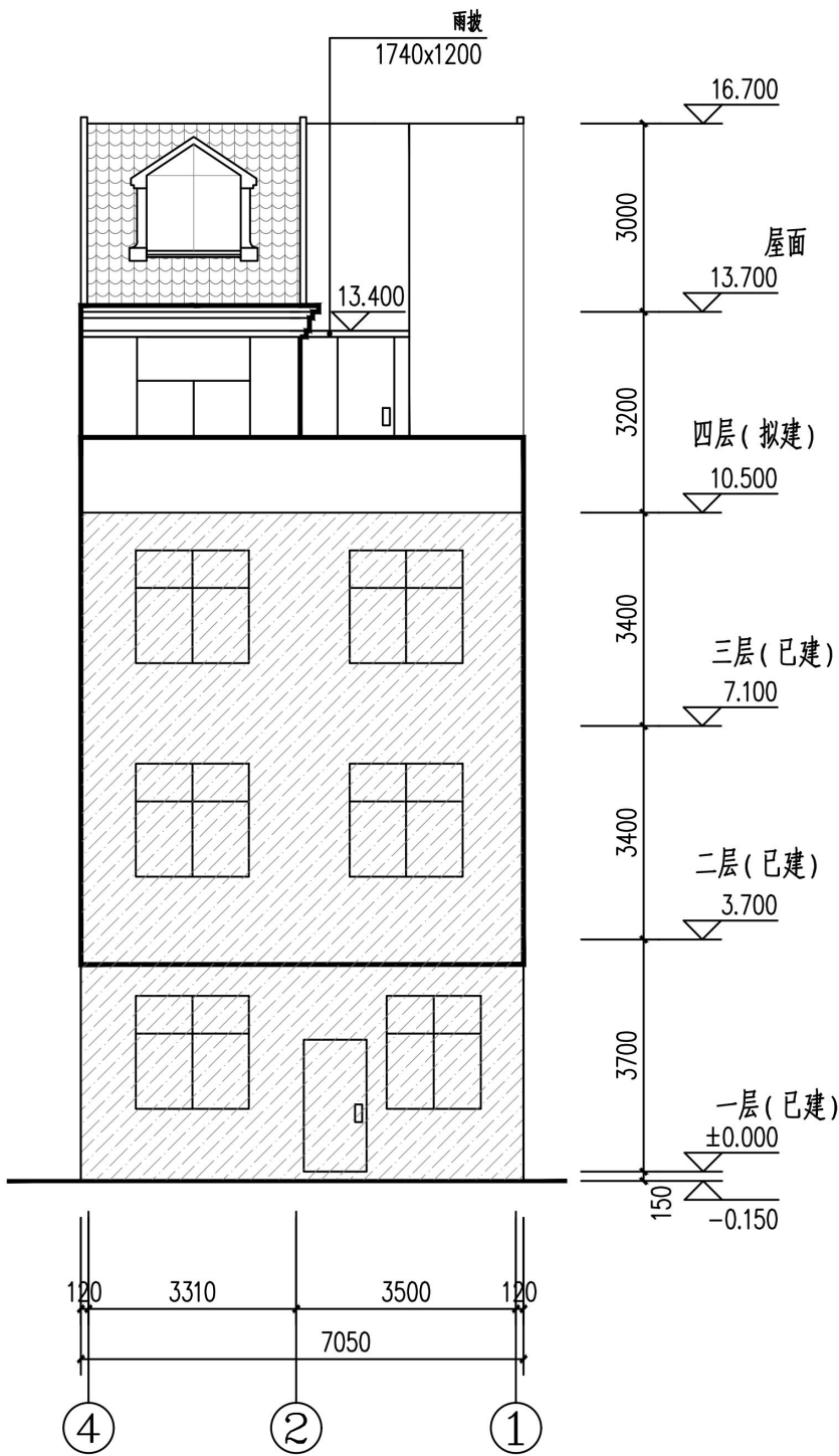
④~①轴立面图 1:100
