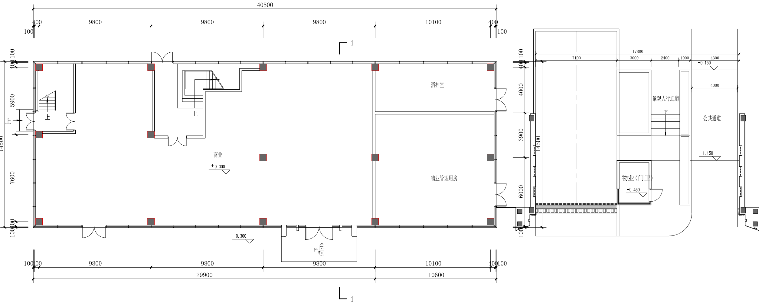
7#楼一层平面图 1:200
