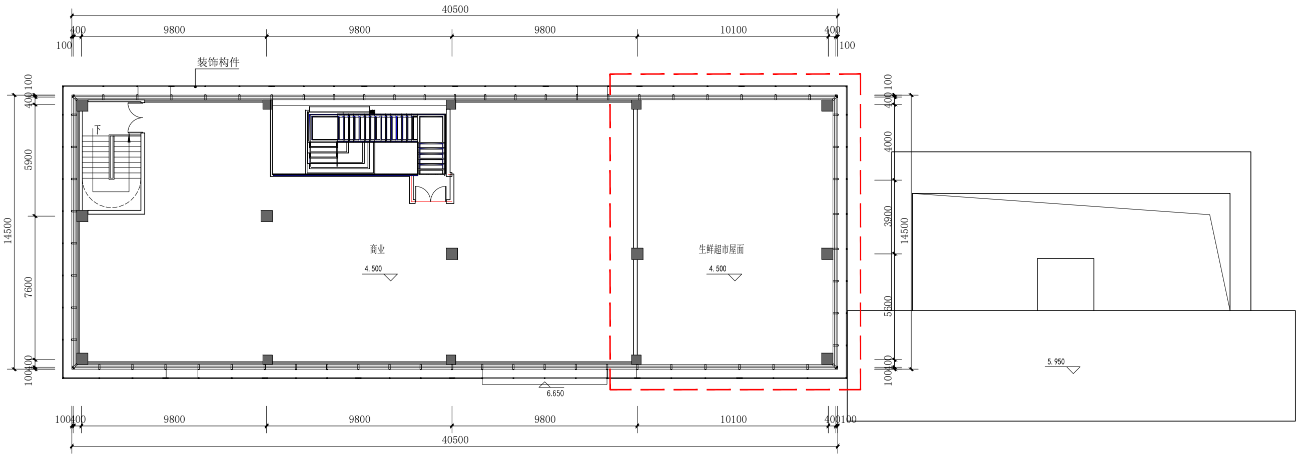
7#楼二层平面图 1:200
