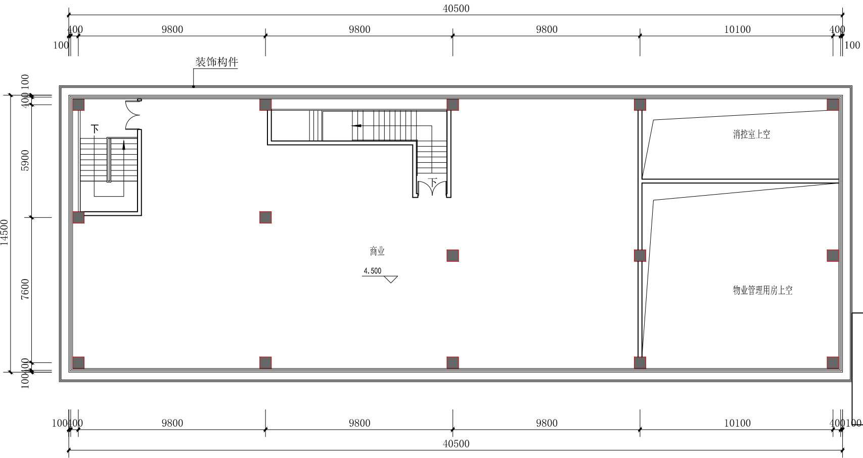
7#楼二层平面图 1:200
