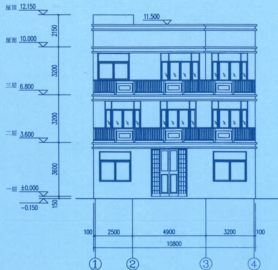
①-④轴立面图 1:100
