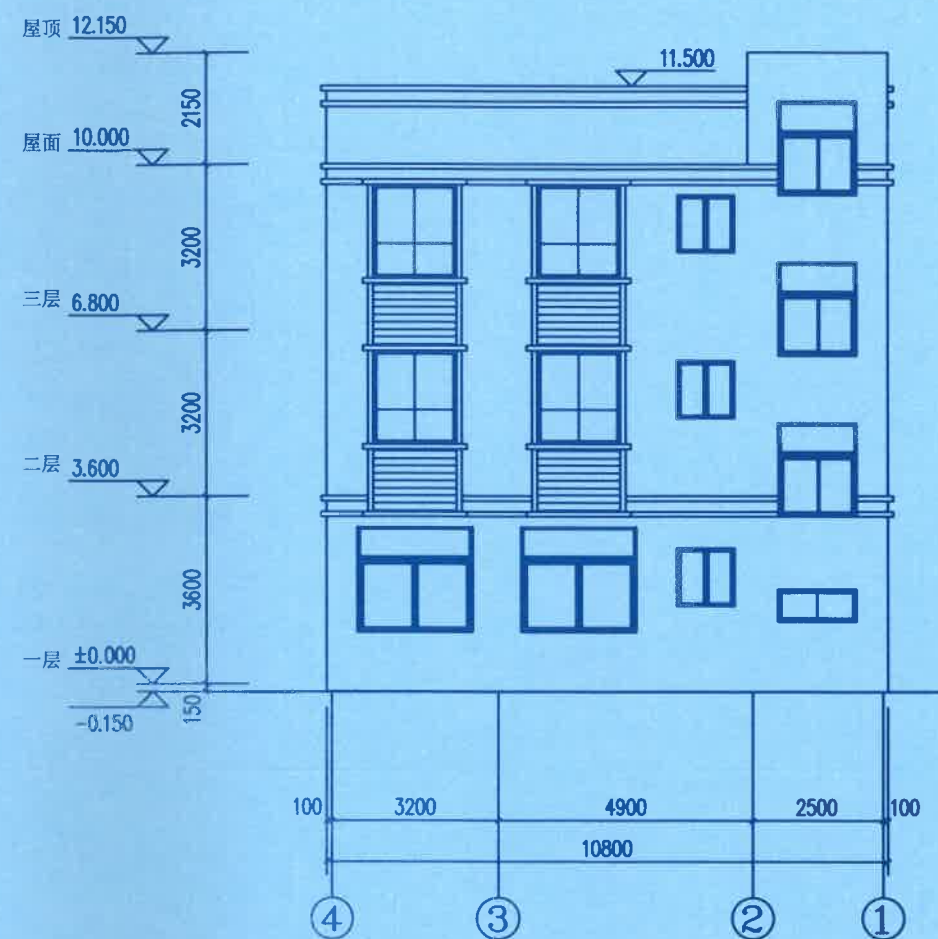
④-①轴立面图 1:100
