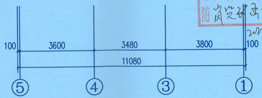
⑤~①轴立面图 1:100
