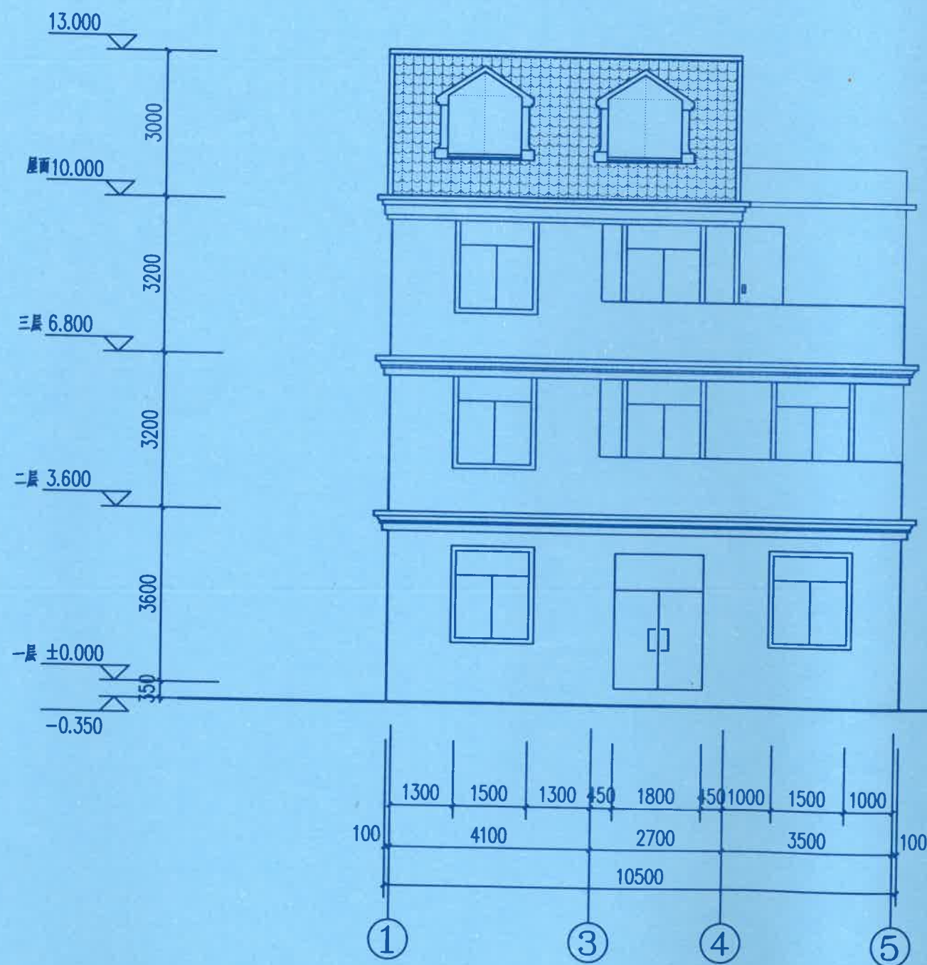
①~⑤轴立面图 1:100
