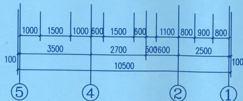
⑤~①轴立面图 1:100
