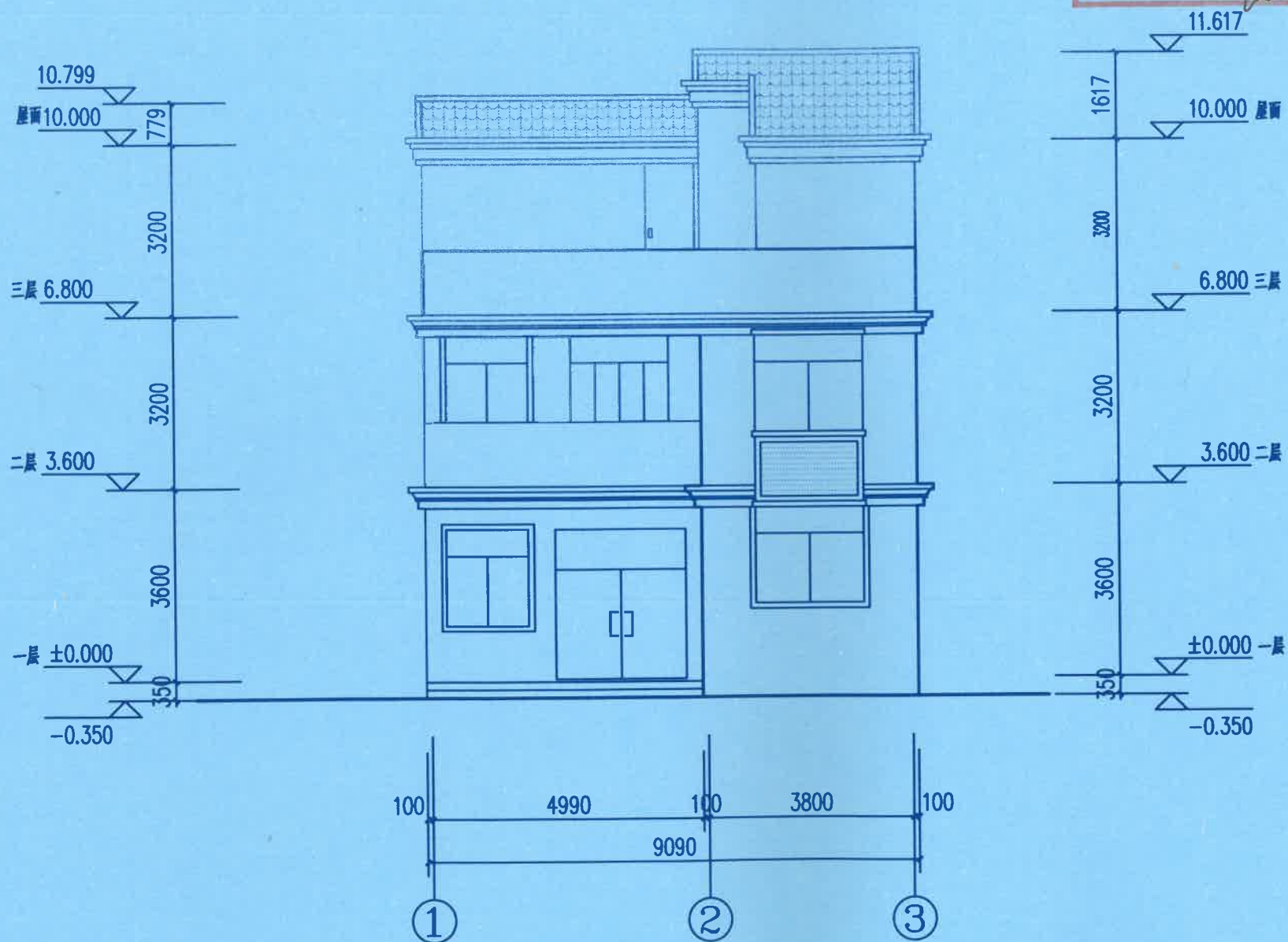
①~③轴立面图 1:100
