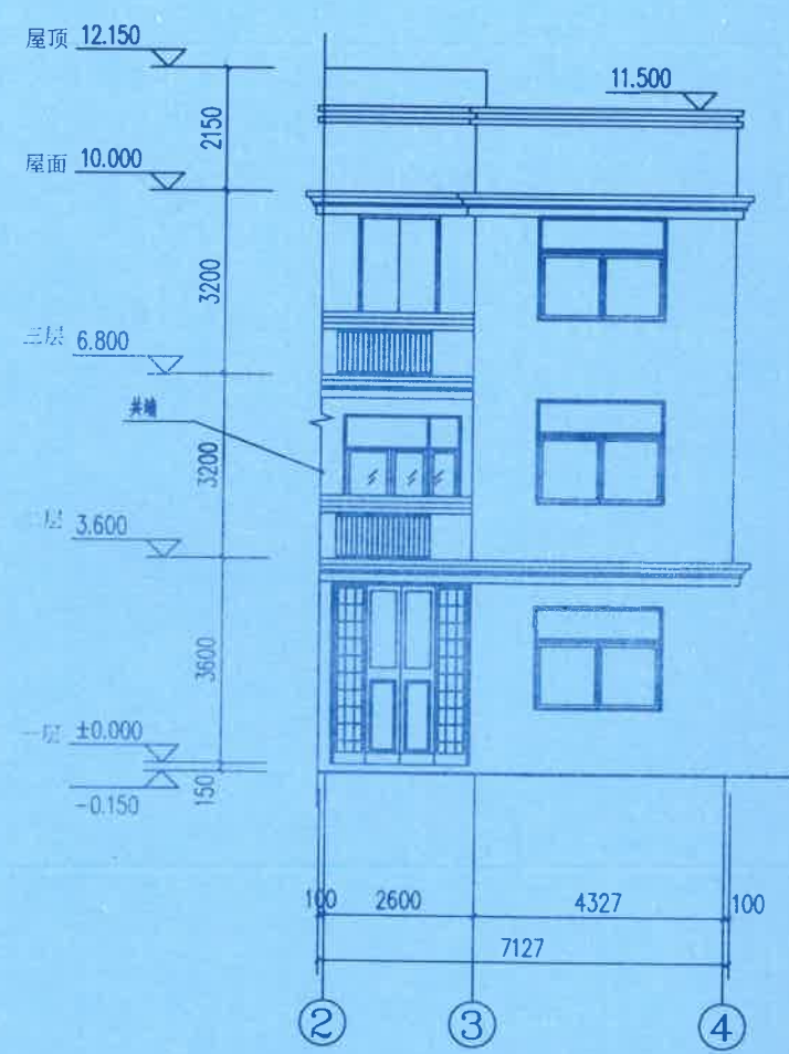
② - ④ 轴立面图 1:100
