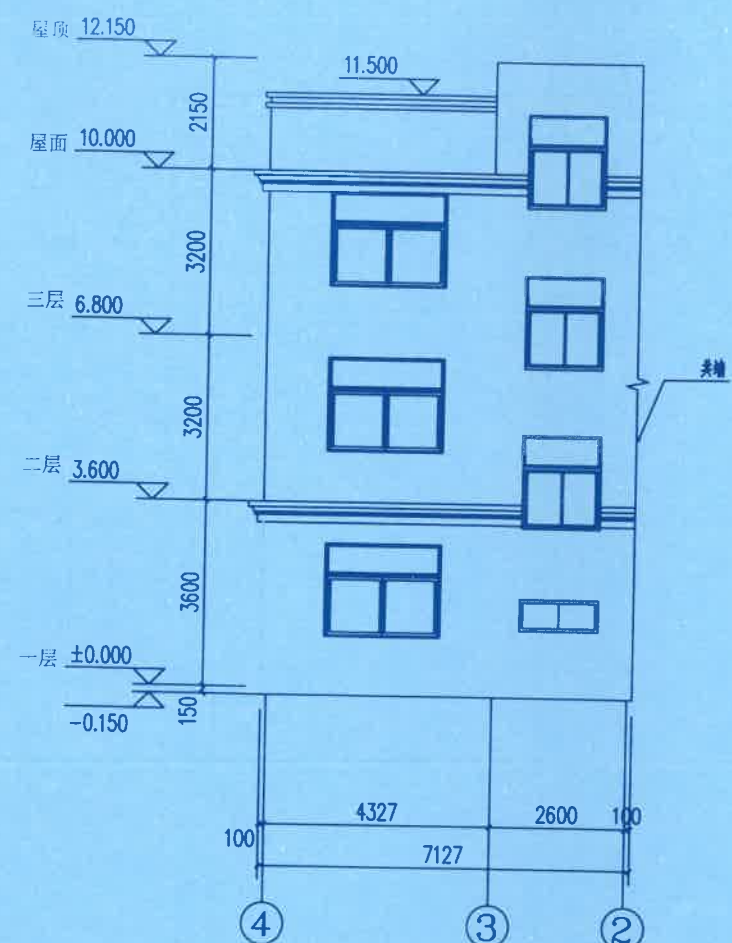
④-②轴立面图 1:100
