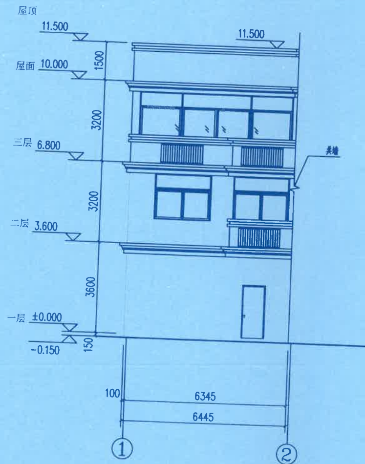
①-② 轴立面图 1:100
