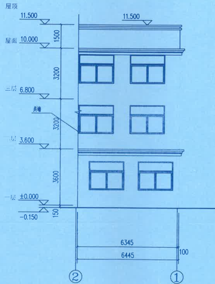
②-①轴立面图 1:100
