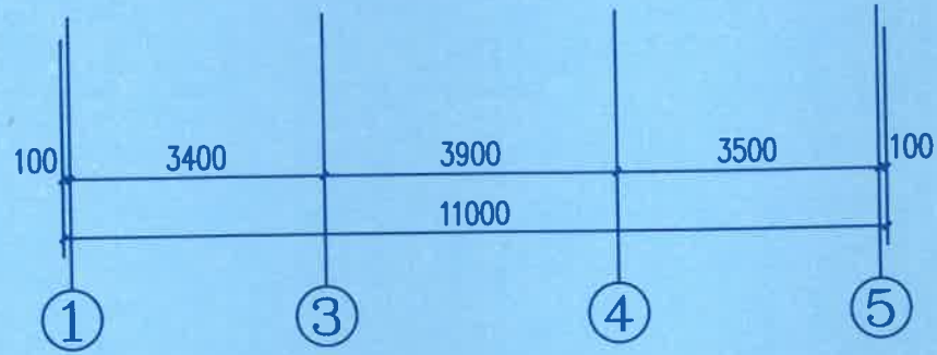
①~⑤轴立面图 1:100
