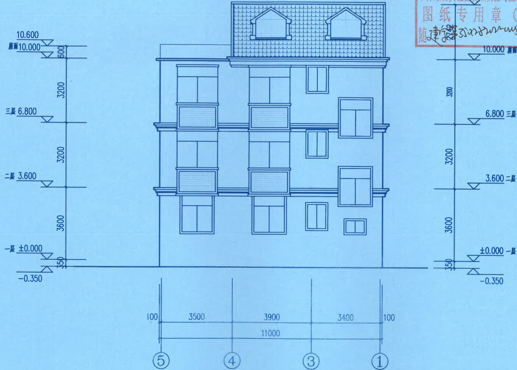
⑤~①轴立面图 1:100
