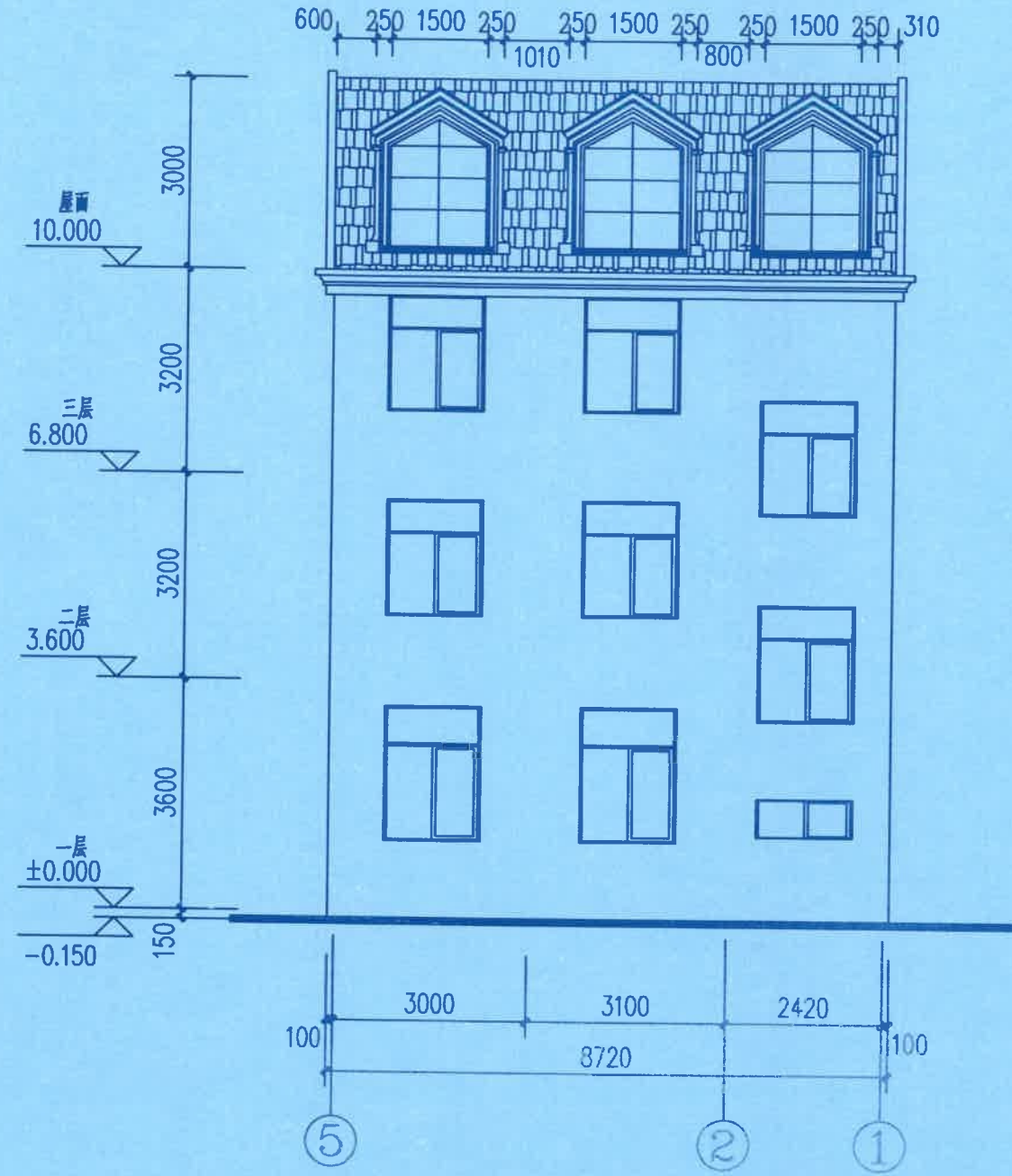
⑤-①轴立面图 1:100
