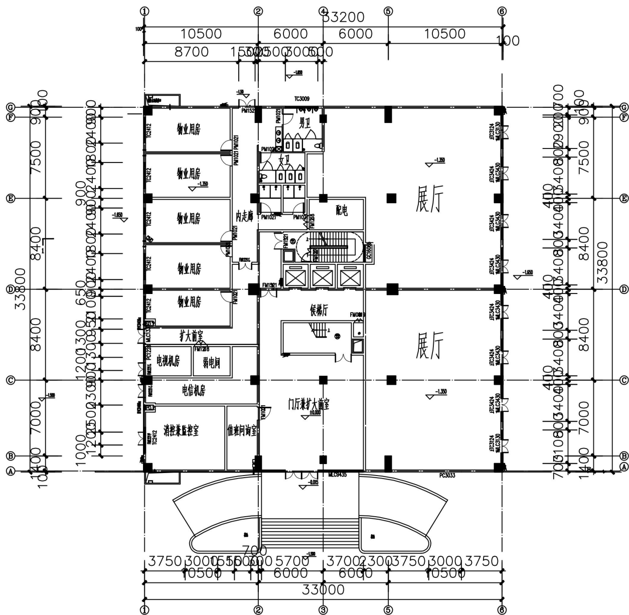
调整后3#楼一层平面图 1:100
