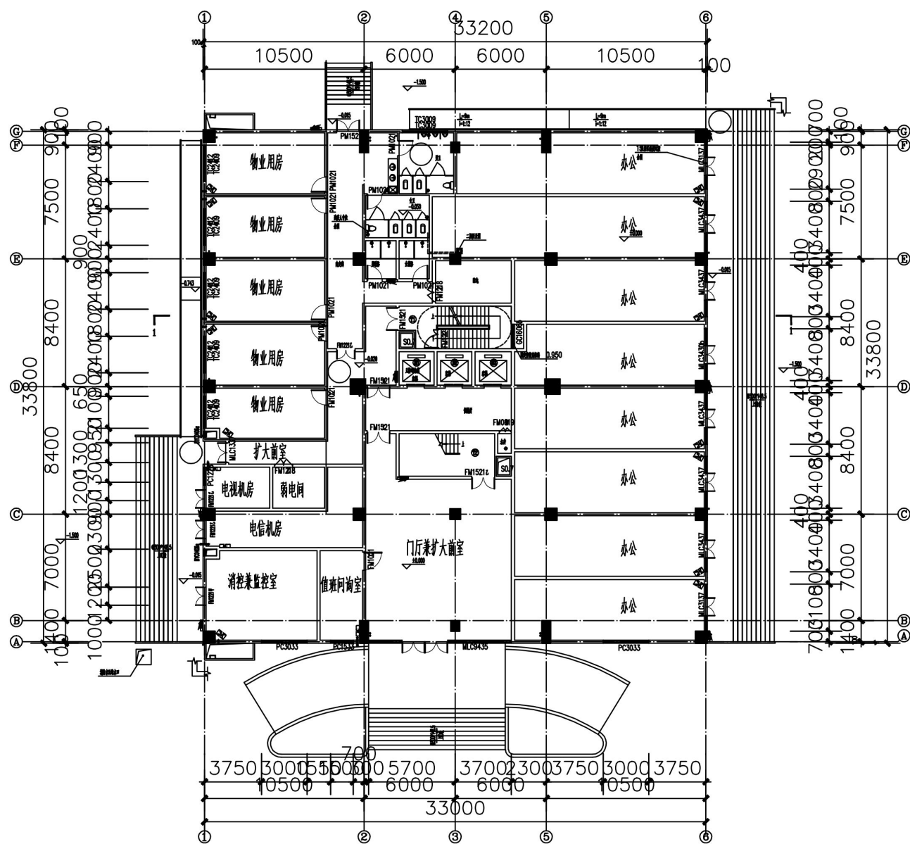
原3#楼一层平面图 1:100
