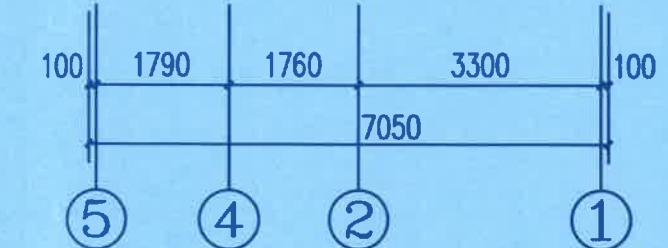
⑤~①轴立面图 1:100
