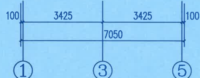
①~⑤轴立面图 1:100 (沿街立面)
