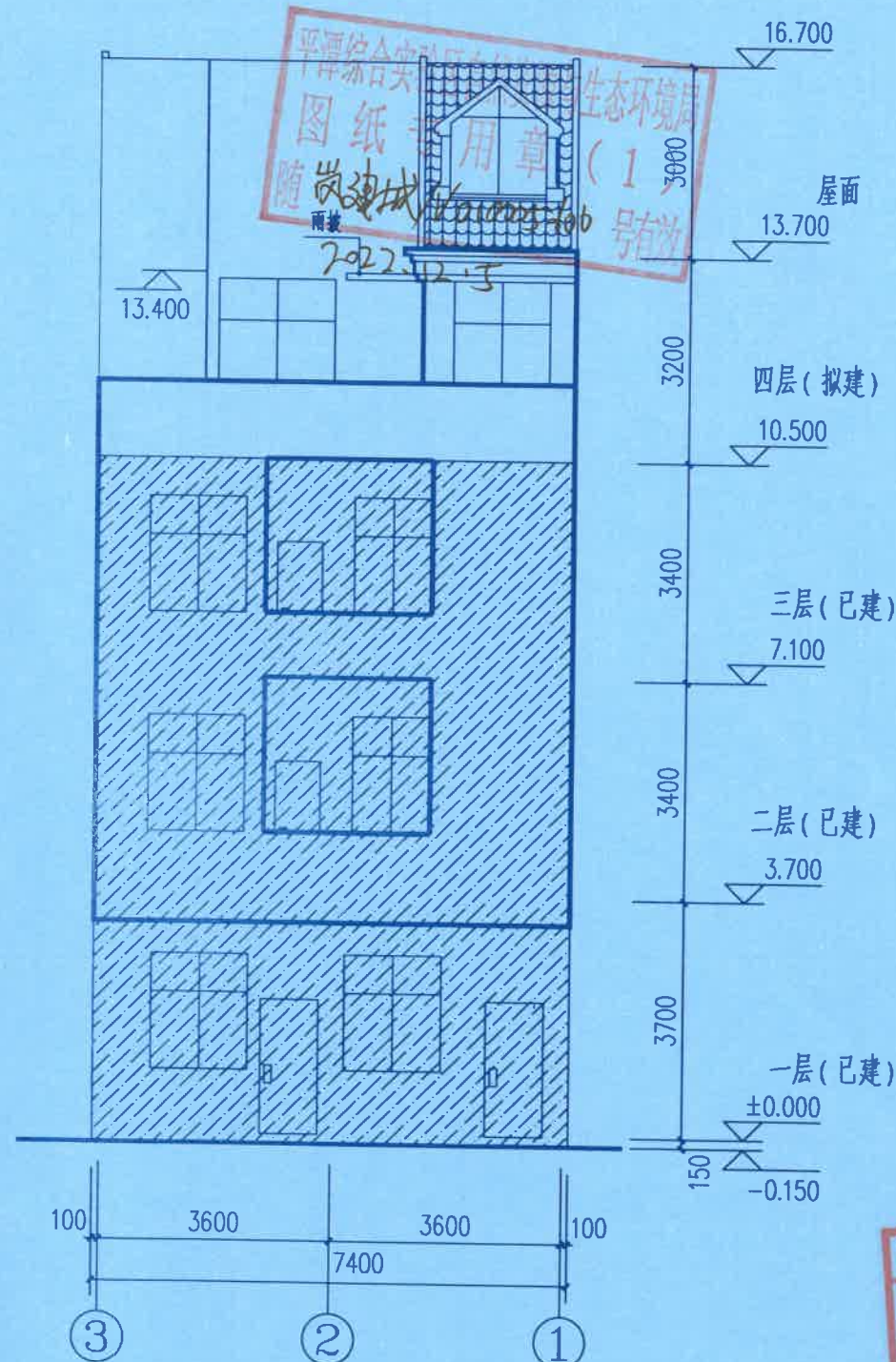
③~①轴立面图 1:100
