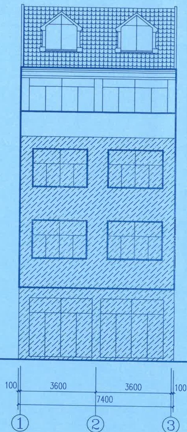
①~③轴立面图 1:100 (沿街面)
