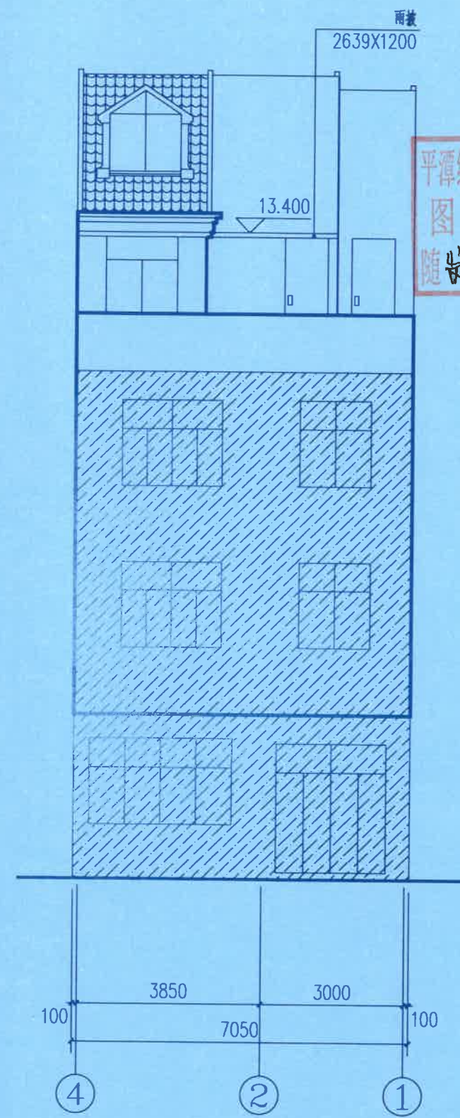
④~①轴立面图 1:100
