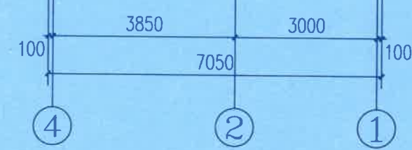
④~①轴立面图 1:100
