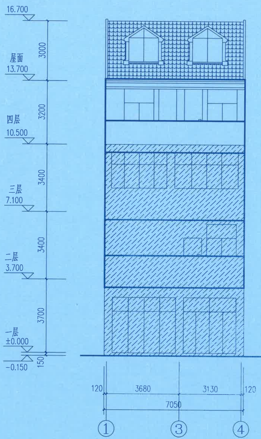
①~④轴立面图 1:100 (沿街面)
