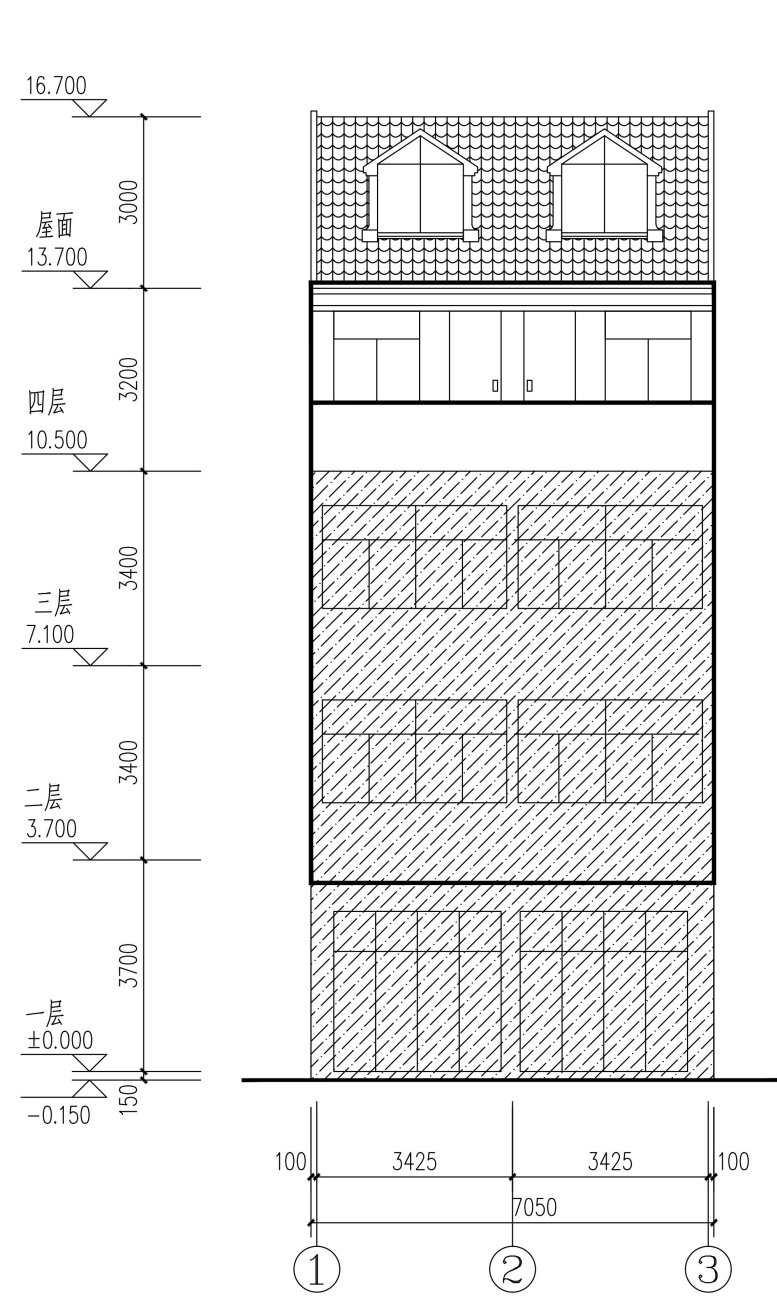
①~③轴立面图 1:100 (沿街面)
