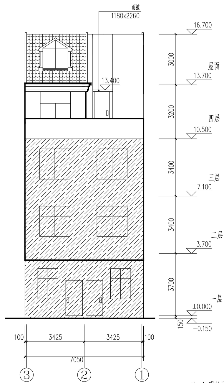
③~①轴立面图 1:100
