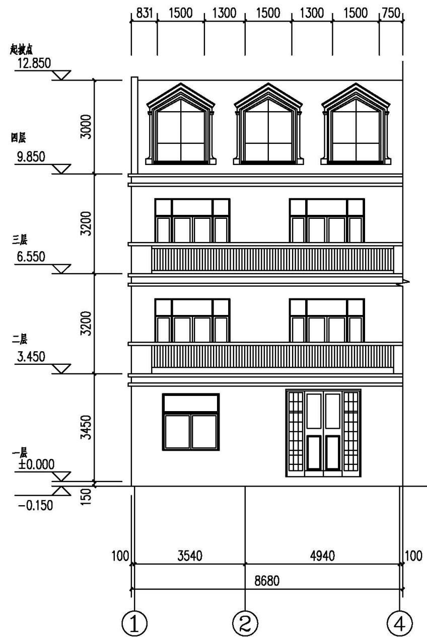
①~④轴立面图 1:100
