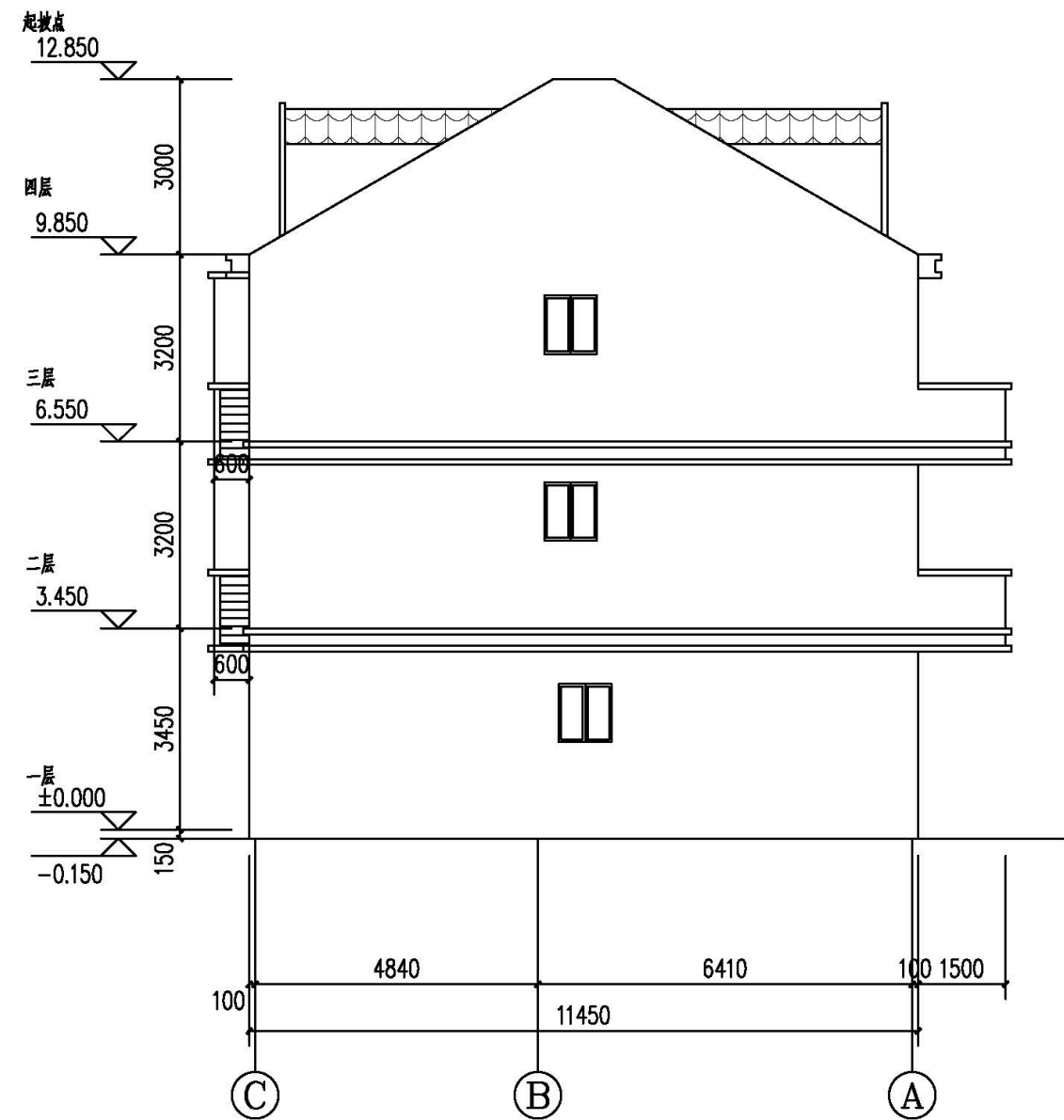
C~A轴立面图 1:100
